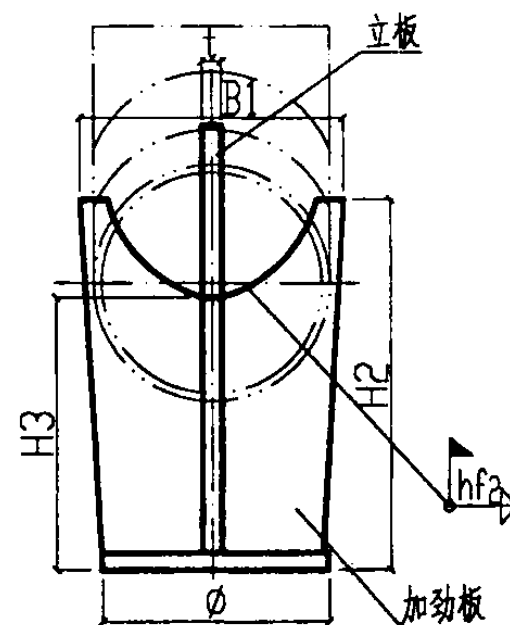
DN200-DN400侧面图
