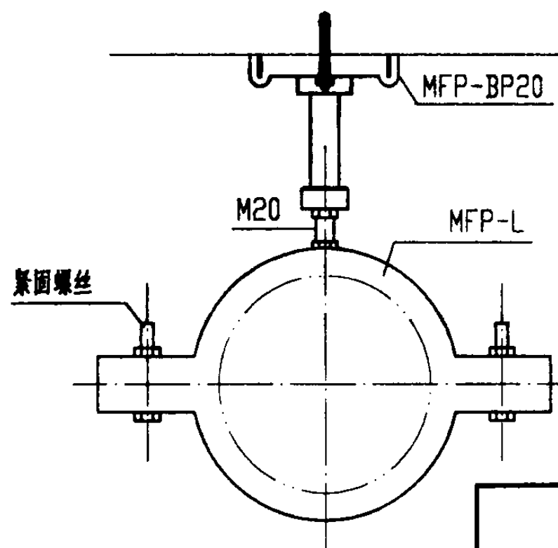
类型2 MFP1a固定支座正立面
