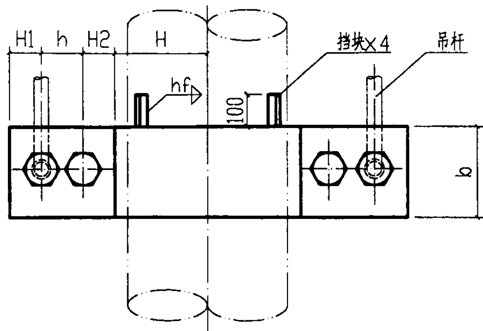
立面图
