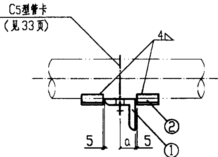
I-I视图
