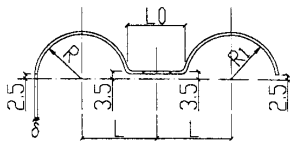
卡板图
