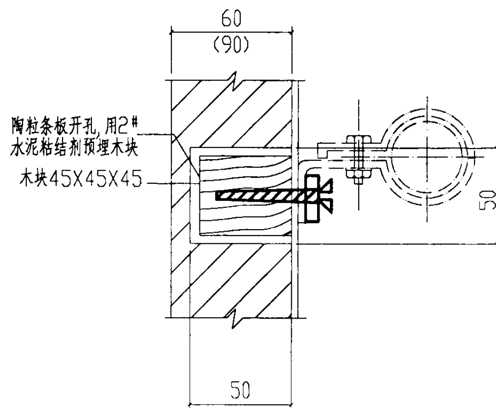
④ 陶粒条板预埋木吊挂件节点
