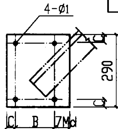
钢板④大样图
