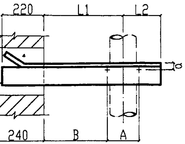
DN50-DN150 立面图
