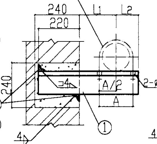
DN150 立面图
