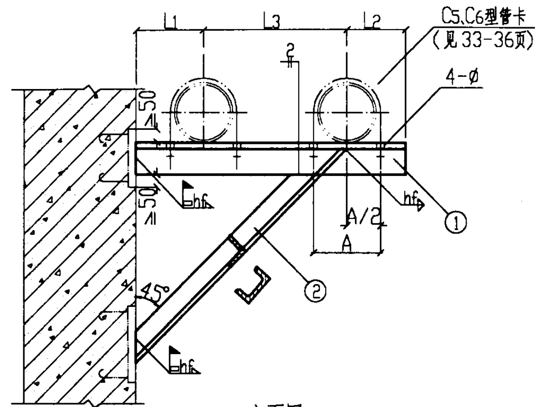
立面图
