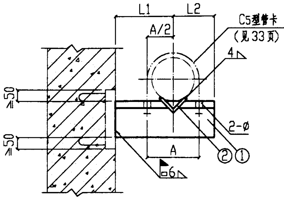
立面图 (平面图)
