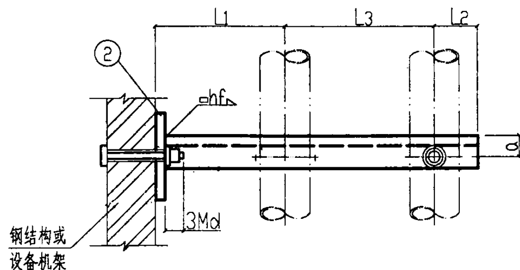
平 面 图
