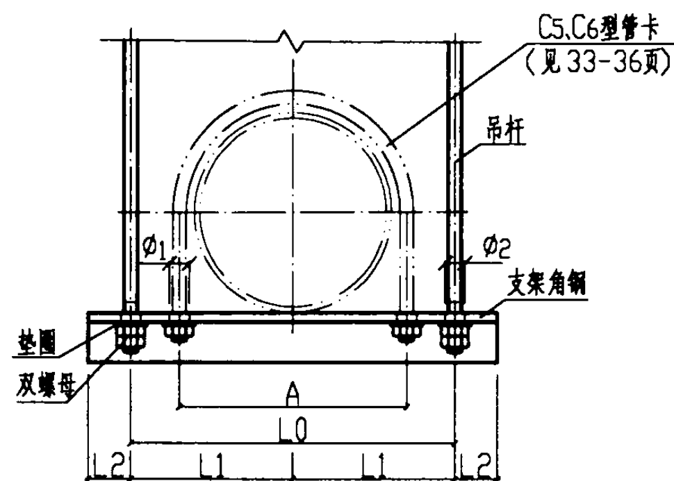
立面图
