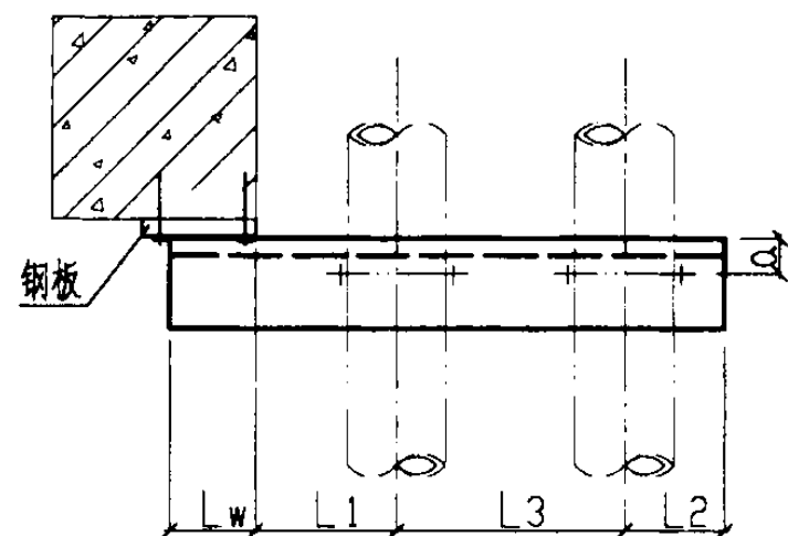
平面图
