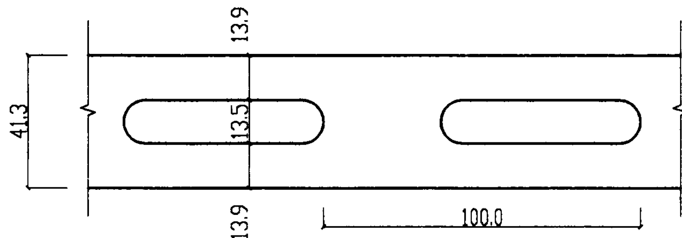
MQ21, MQ41, MQ72平面图
