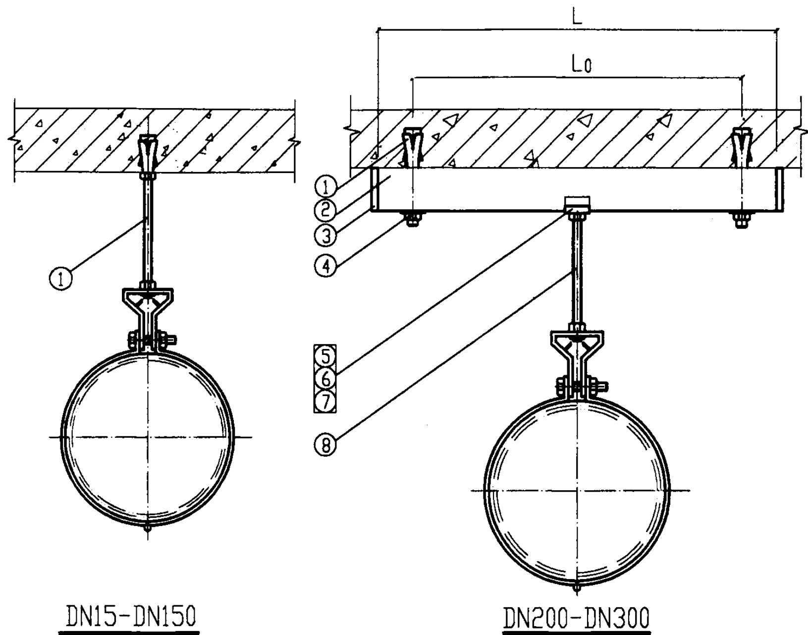
立面图
