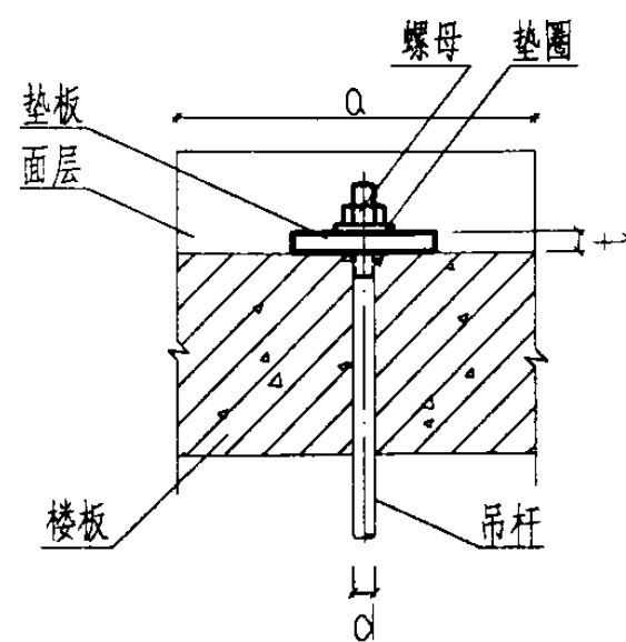
立面图
