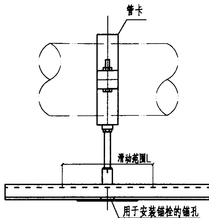
滑动支座MSG1.0侧立面
