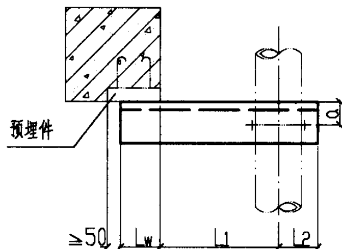
平面图
