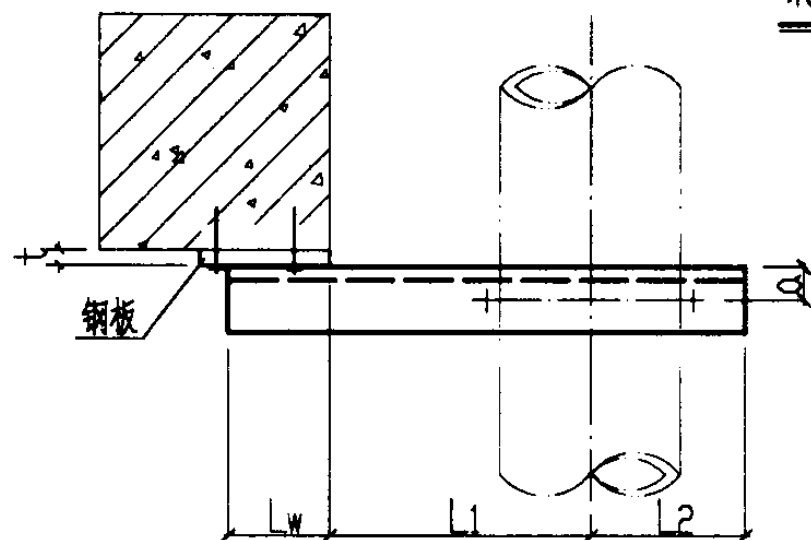
平面图
