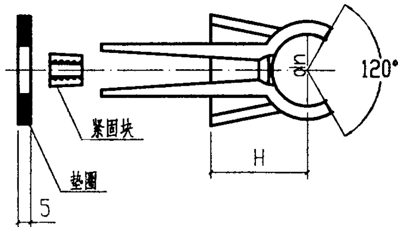
墙卡(二)
