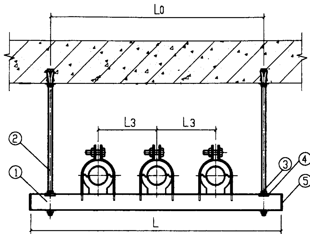
立面图(保温)
