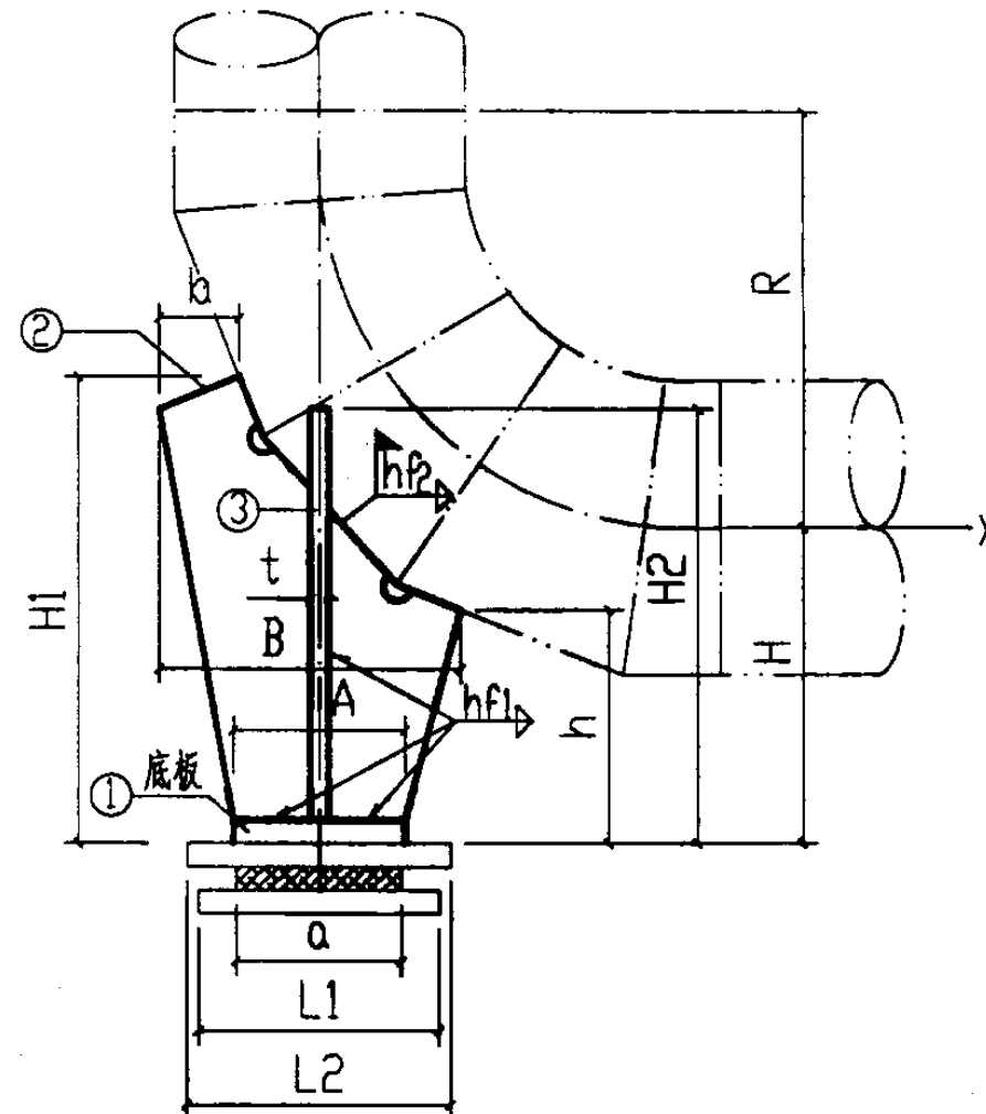
立面图
