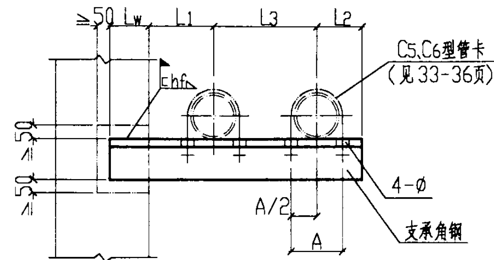
立面图
