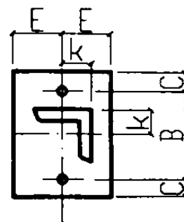
钢板大样图
