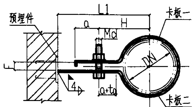
I型支架平面图
