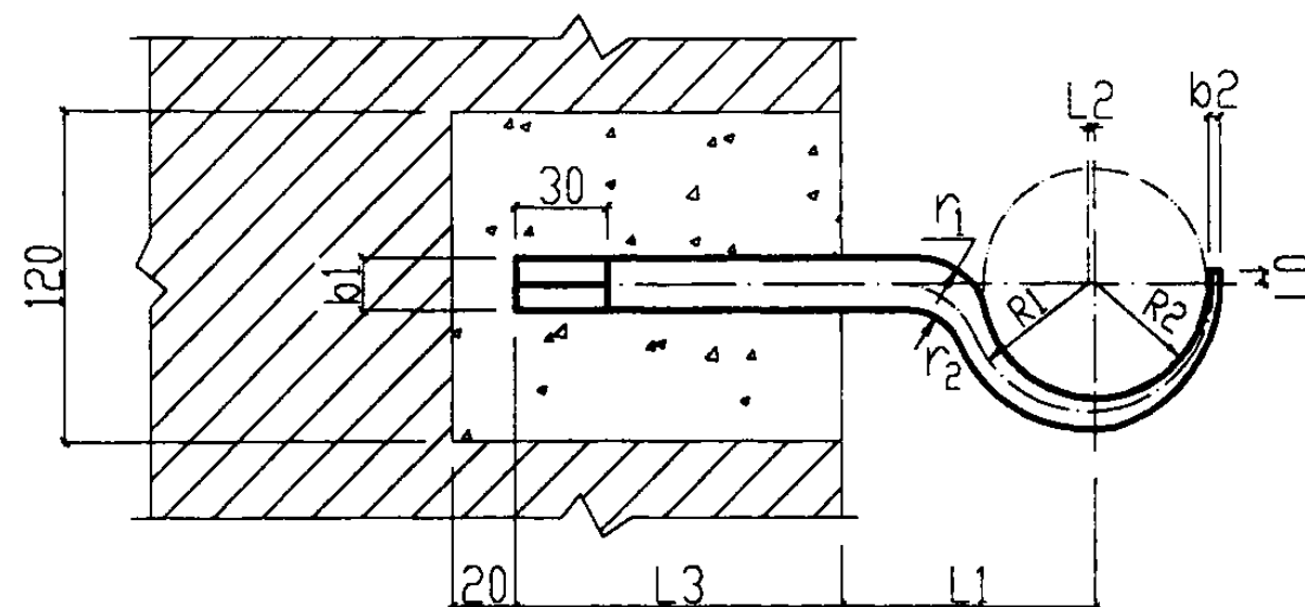
立面图
