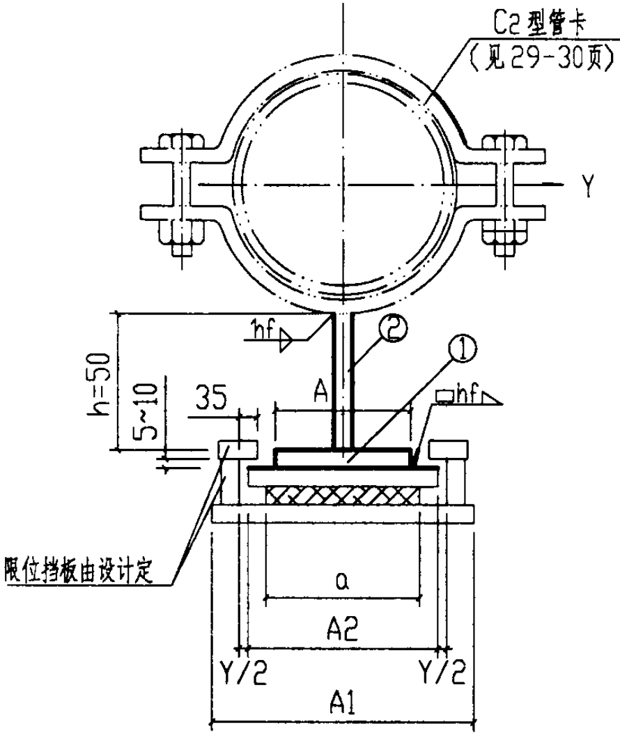
侧面图
