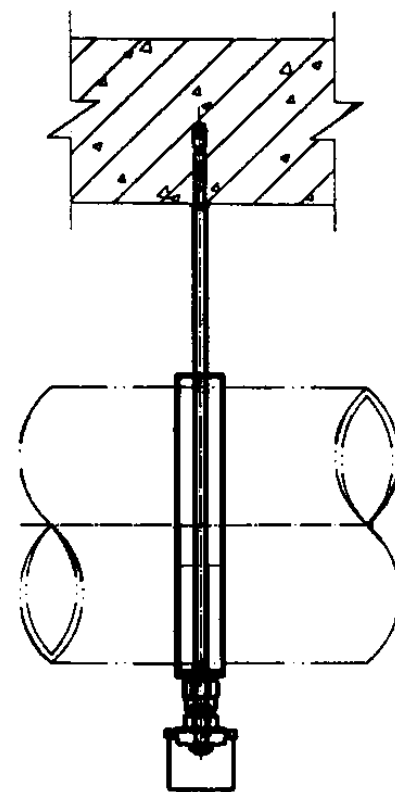
侧面图
