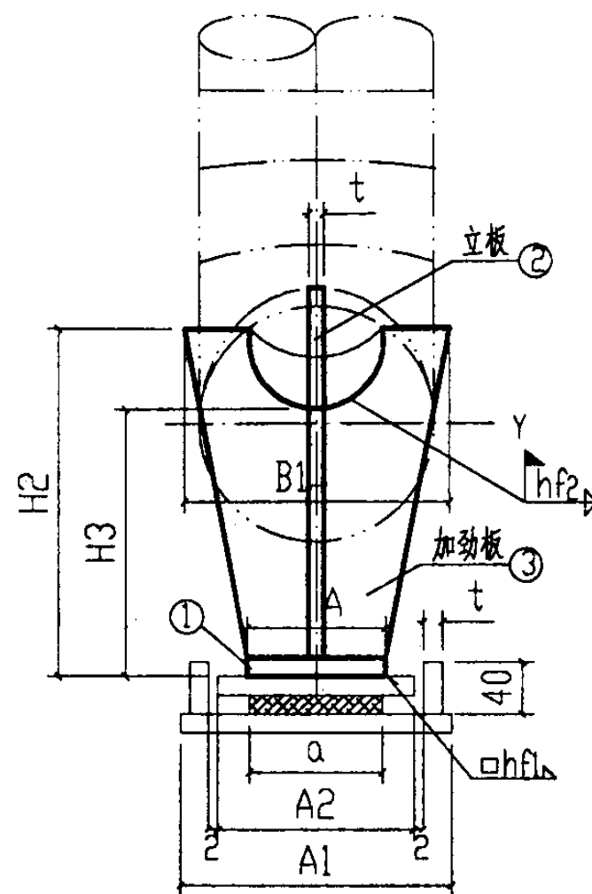
侧面图
