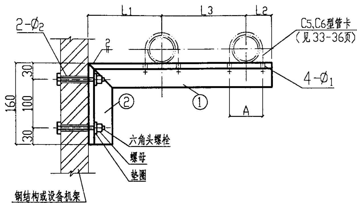
立面图
