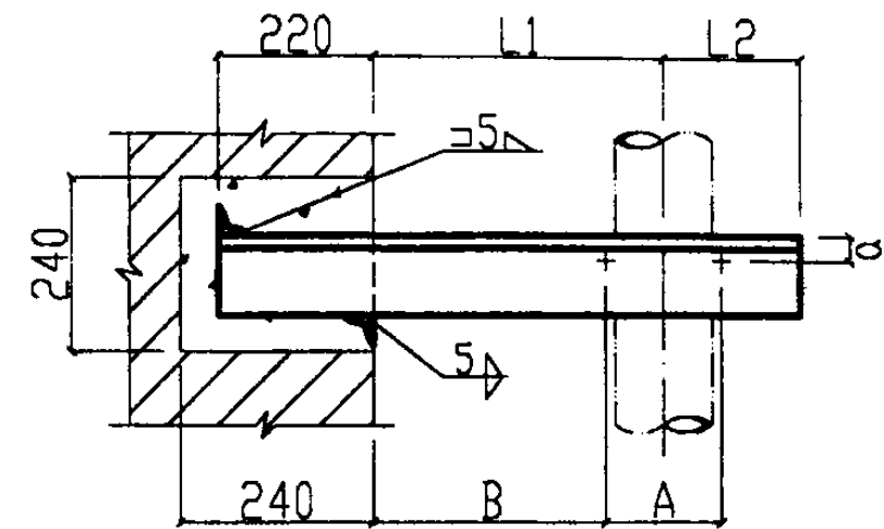
DN200-DN400 立面图
