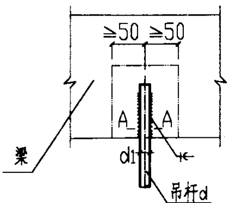
立面图
