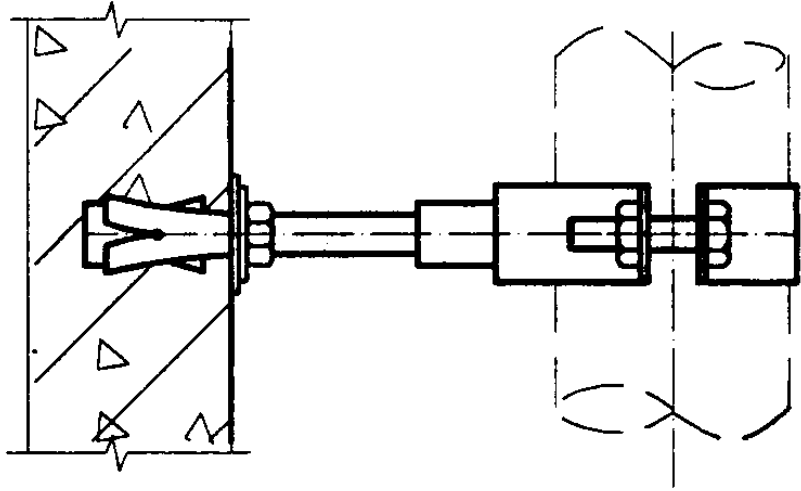
立 面 图
