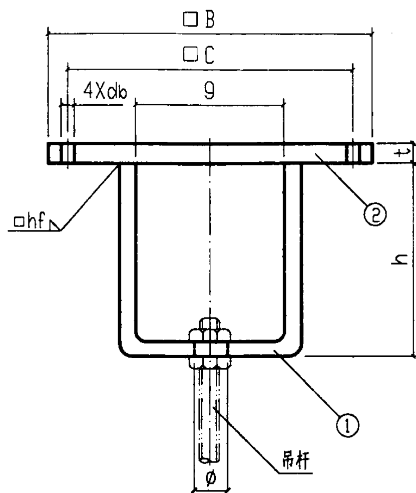
立面图
