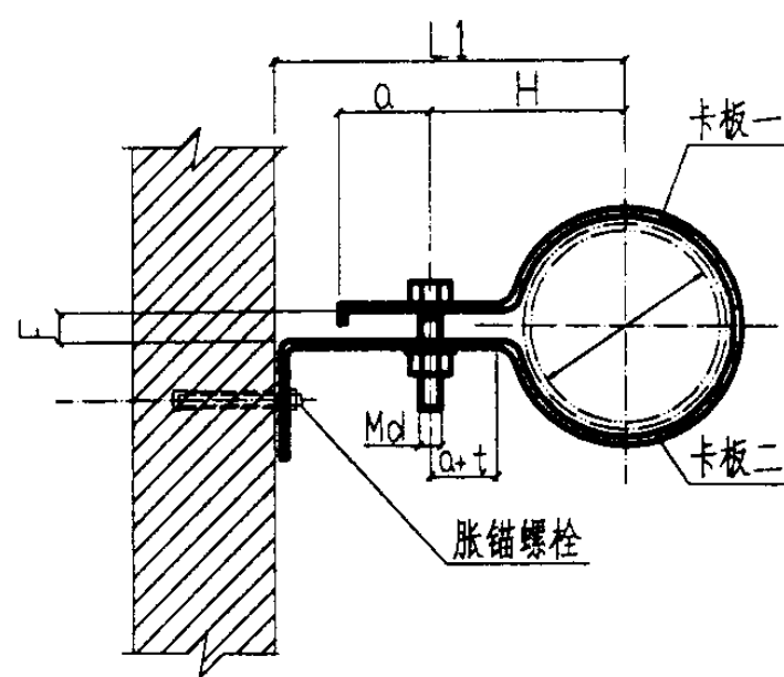
立面图
