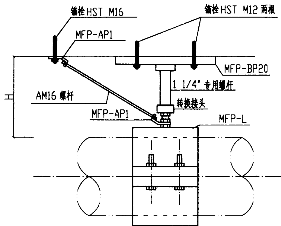
类型1 MFP1固定支座侧立面
