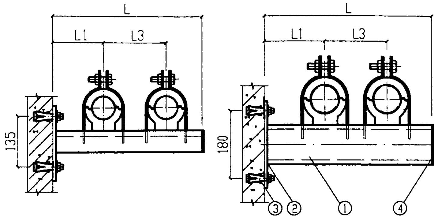
立面图
