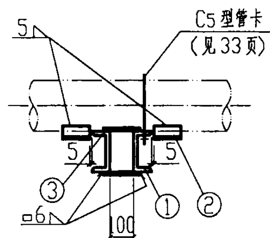
I-I 视图
