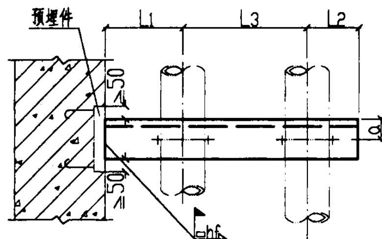
平面图
