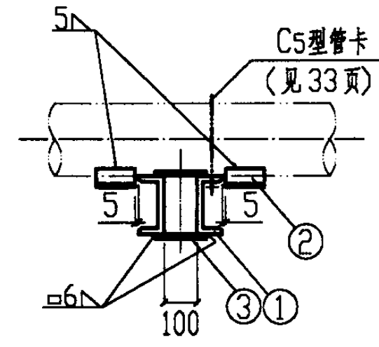
I-I视图
