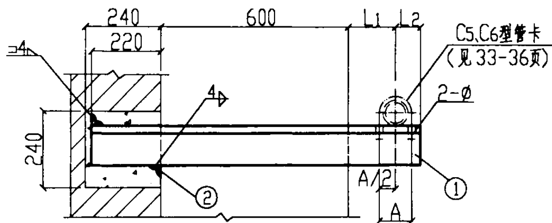
立面图
