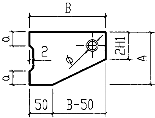
吊板大样
