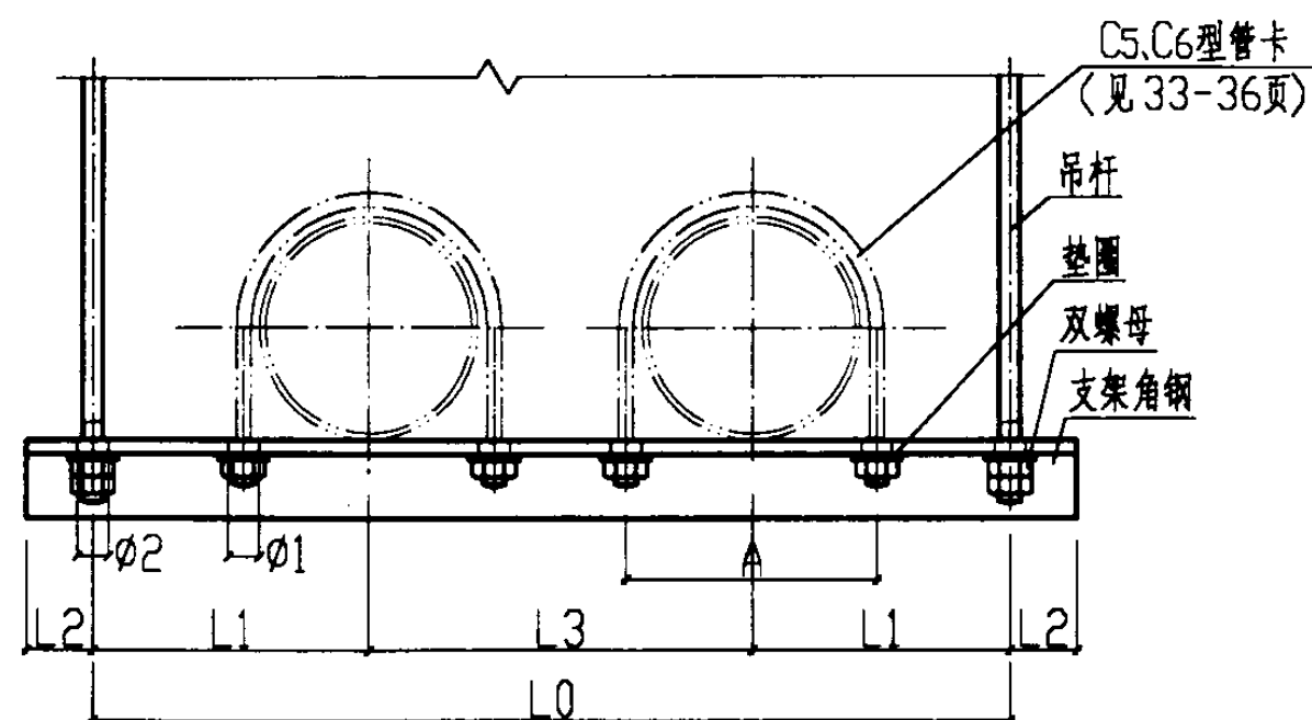
立面图
