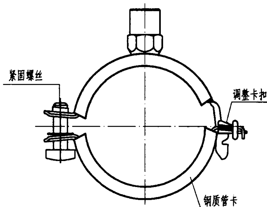
类型7 MPN-S
