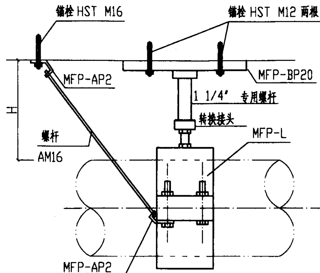
类型3 MFP2固定支座侧立面
