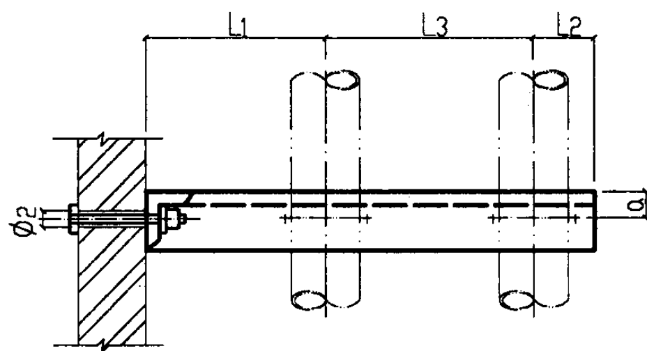
平面图
