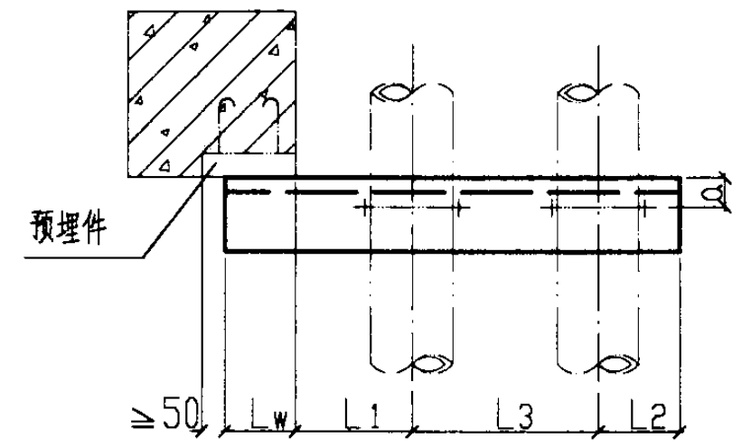
平面图
