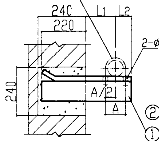
DN15-DN125 立面图
