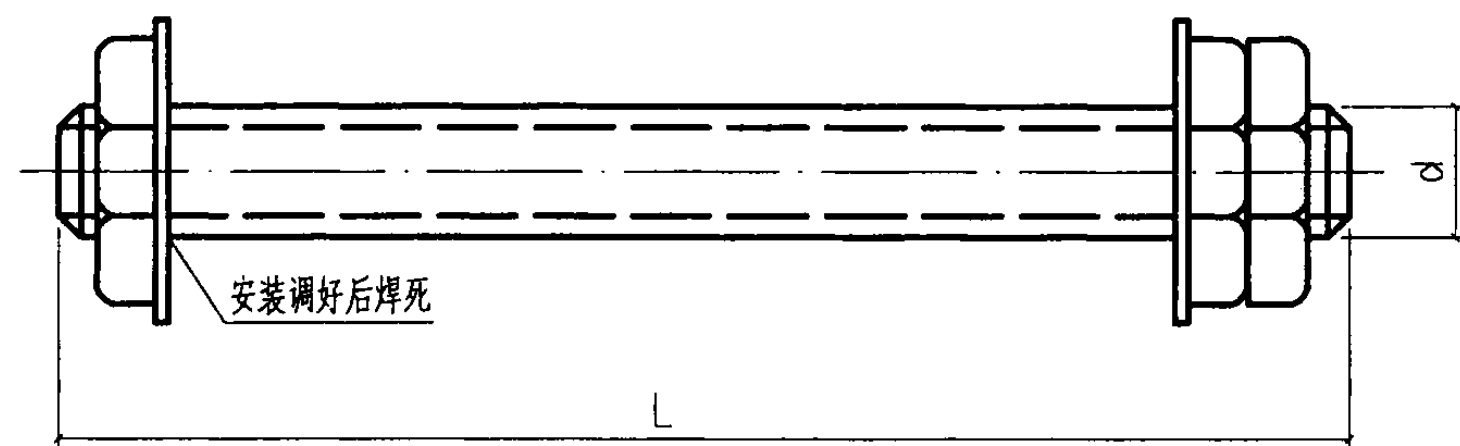
全螺纹吊杆
