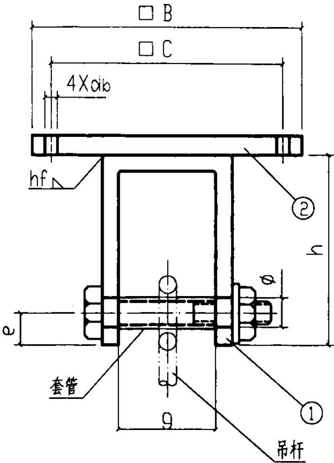
立面图
