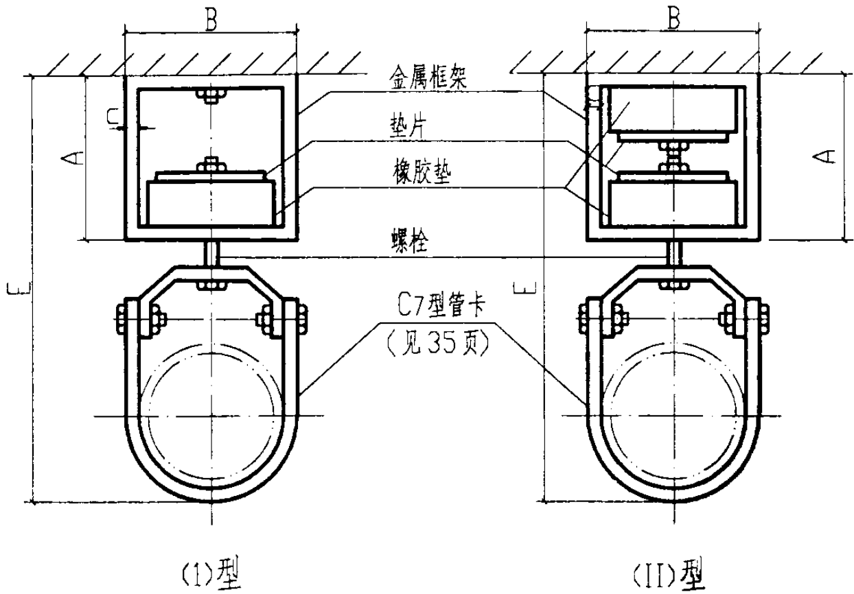
橡胶弹性吊架结构示意图
