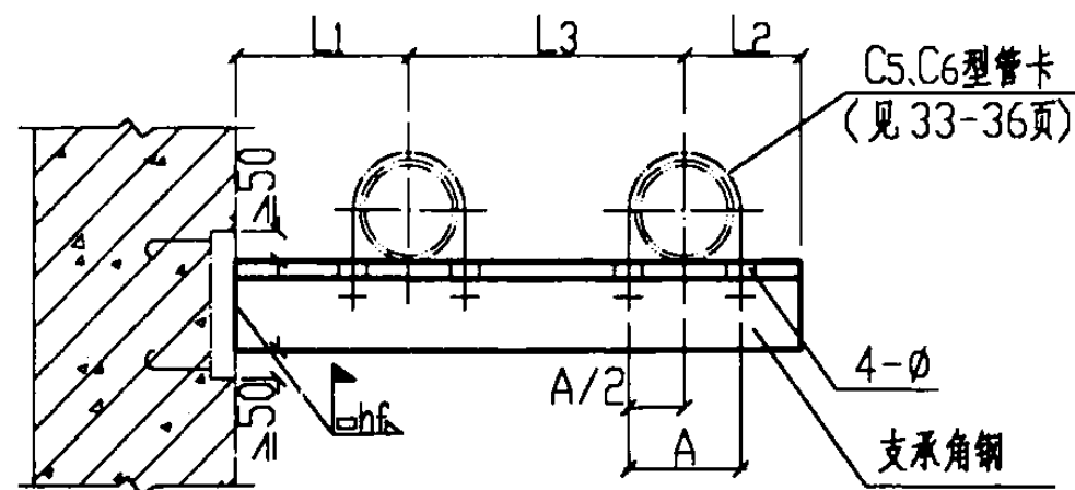
立面图
