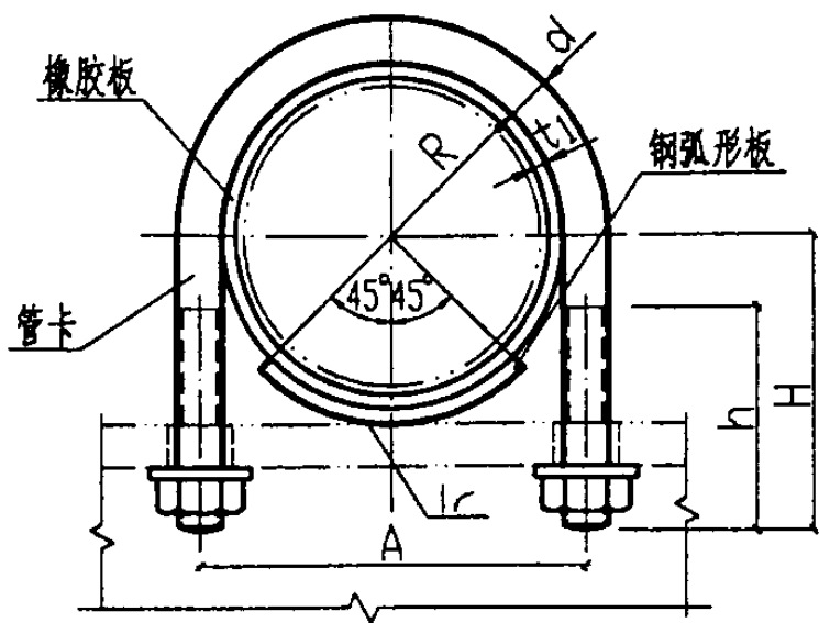
立面图
