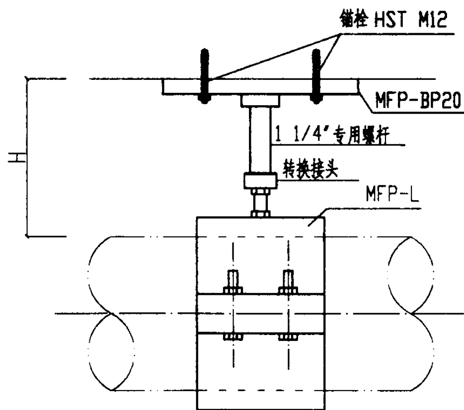
类型2 MFP1a固定支座侧立面
