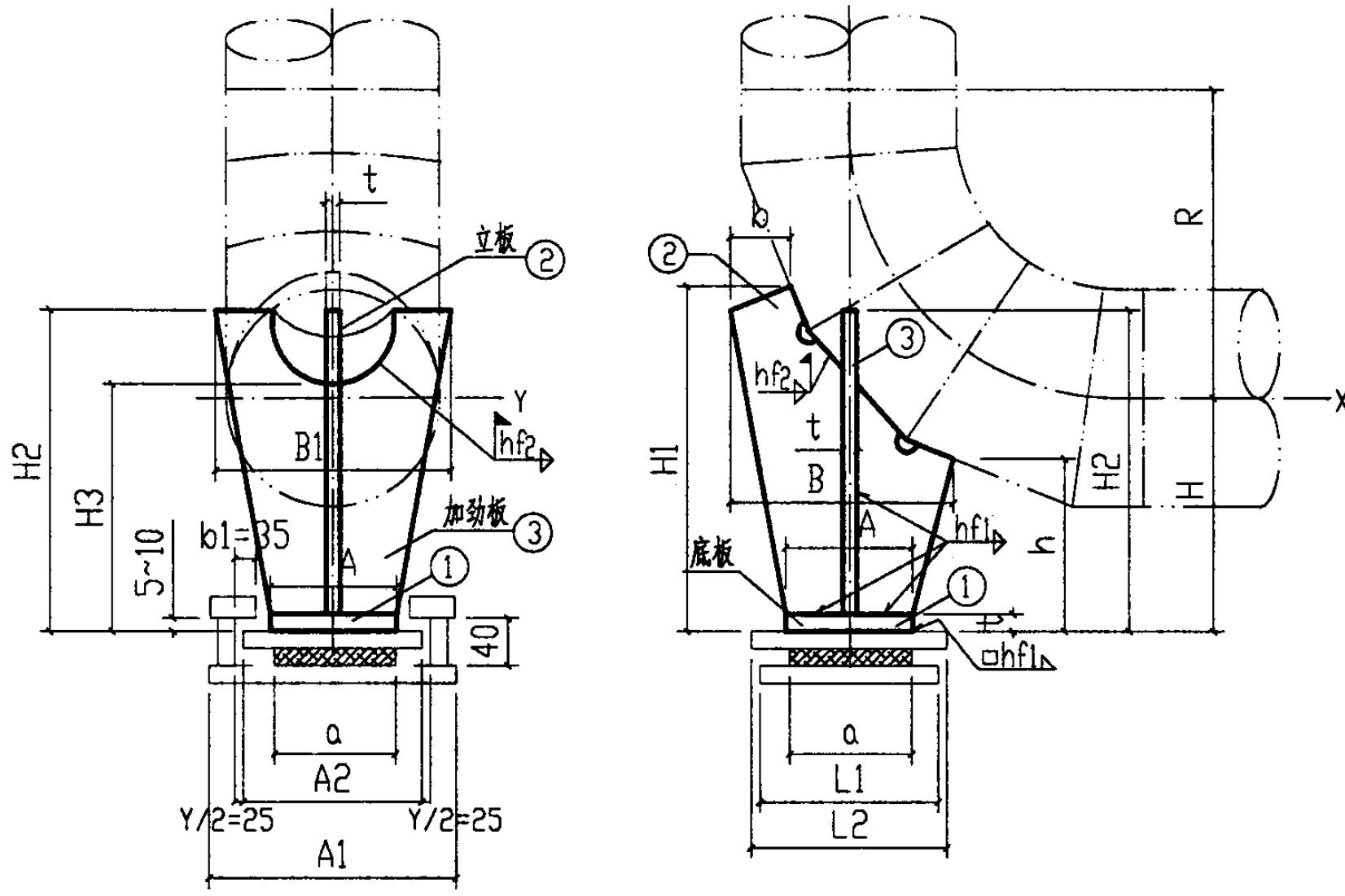
侧面图
