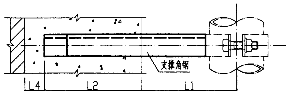
立面图
