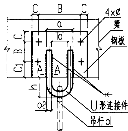
立面图
