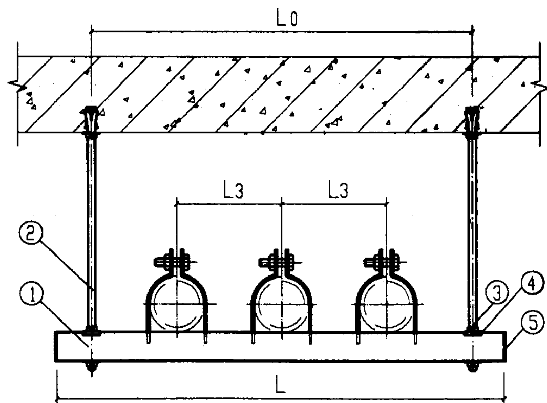
立面图(不保温)
