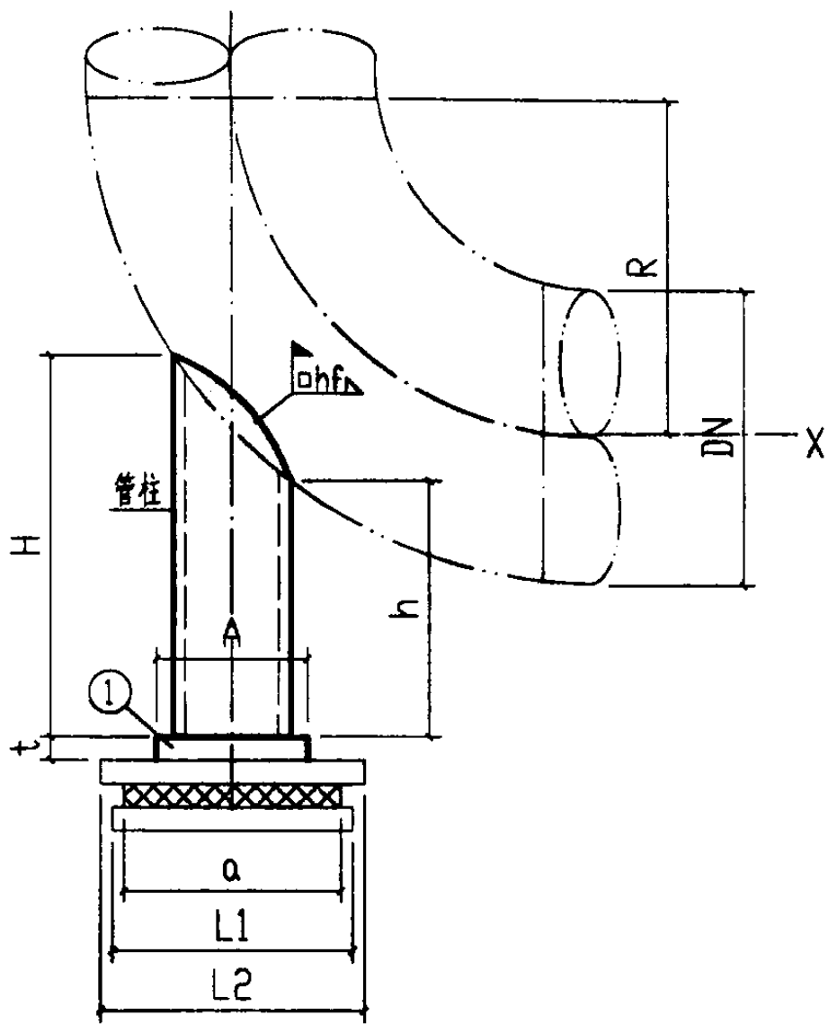
立面图
