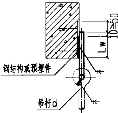
侧面图
