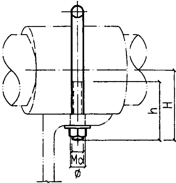
侧面图
