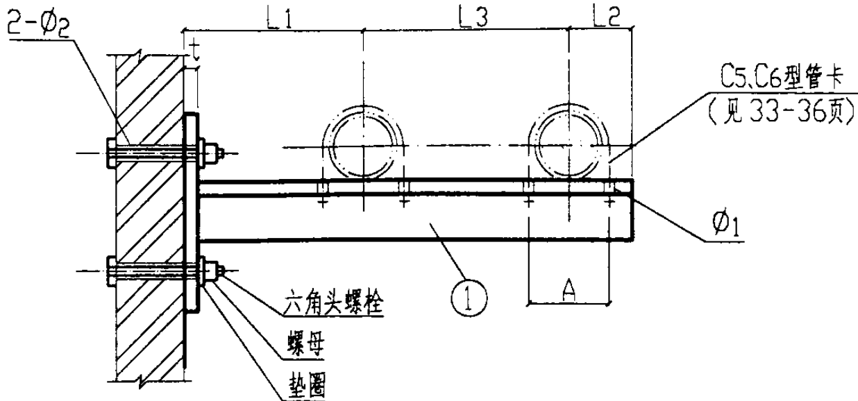
立 面 图
