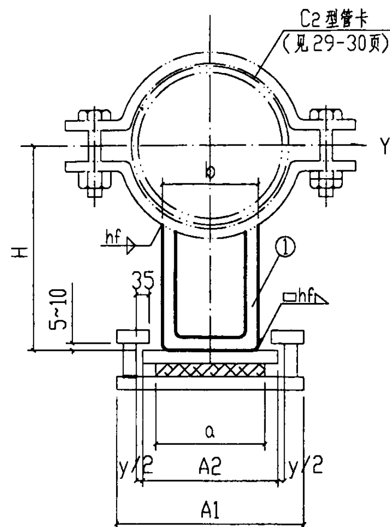
侧面图
