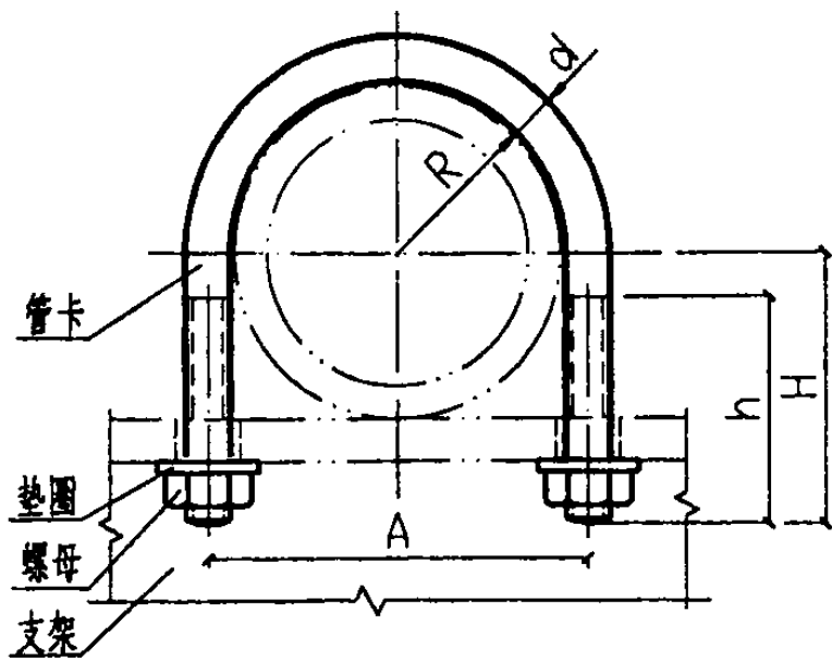
立面图
