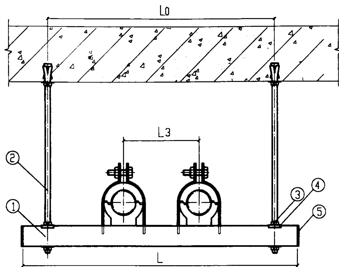
立面图(保温)
