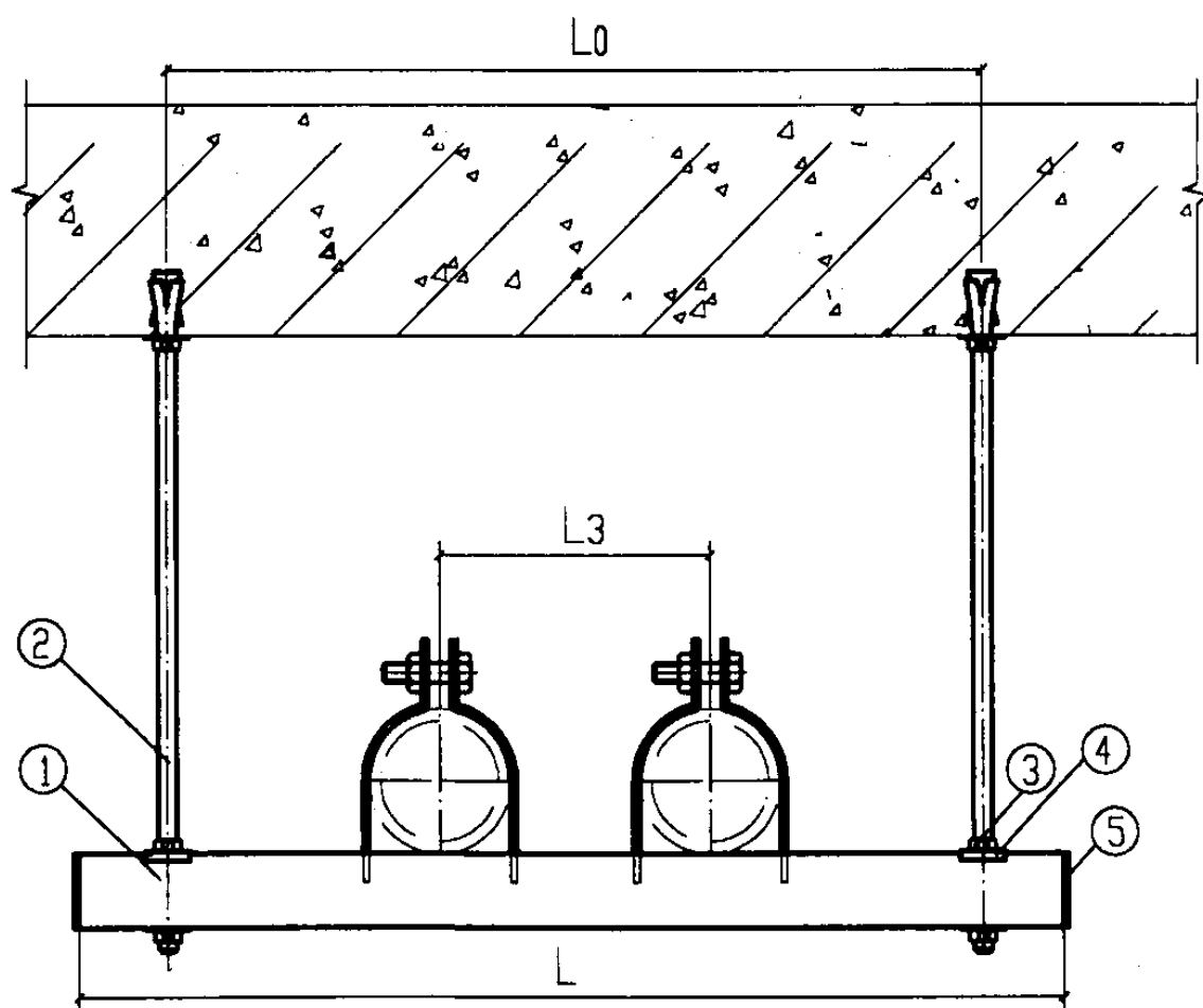
立面图(不保温)
