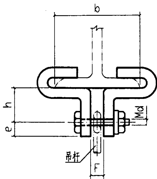
工字钢梁夹
