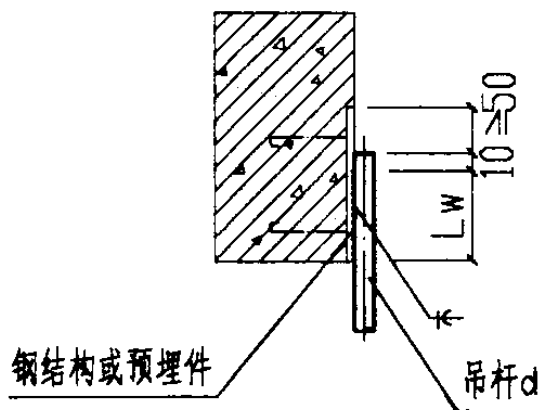
侧面图
