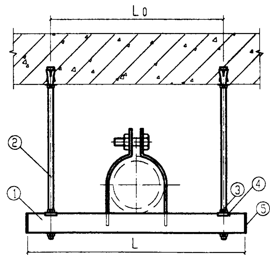
立面图(不保温)
