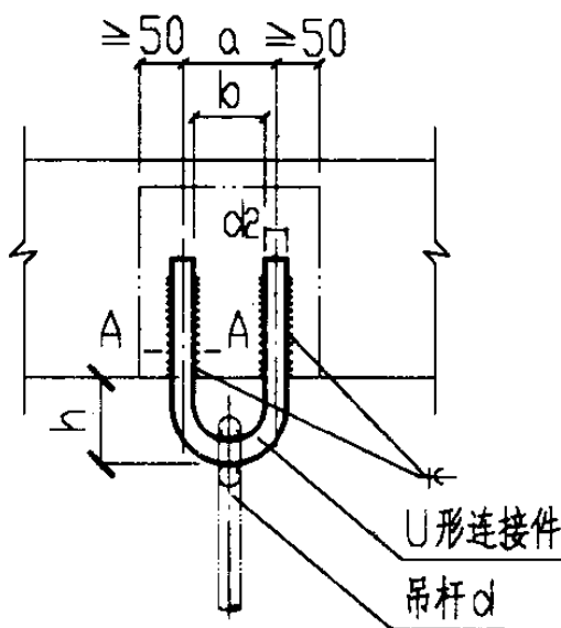
立面图
