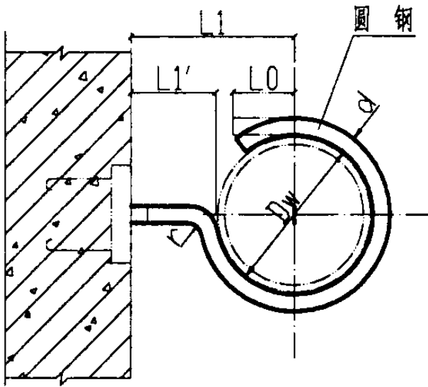
I型平面图
