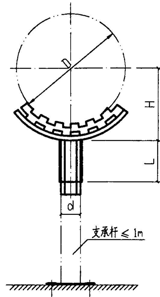
立视图
