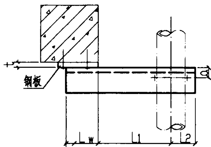
平面图
