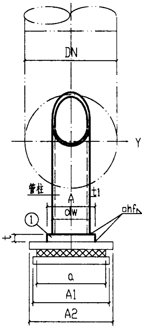
侧面图
