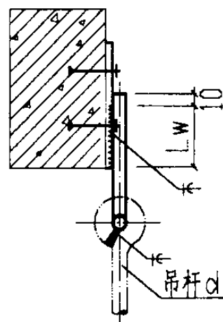
侧面图
