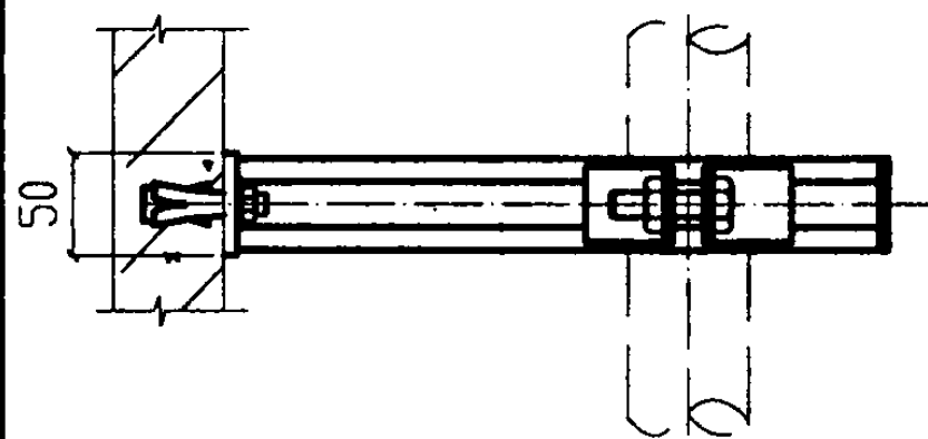
平面图
