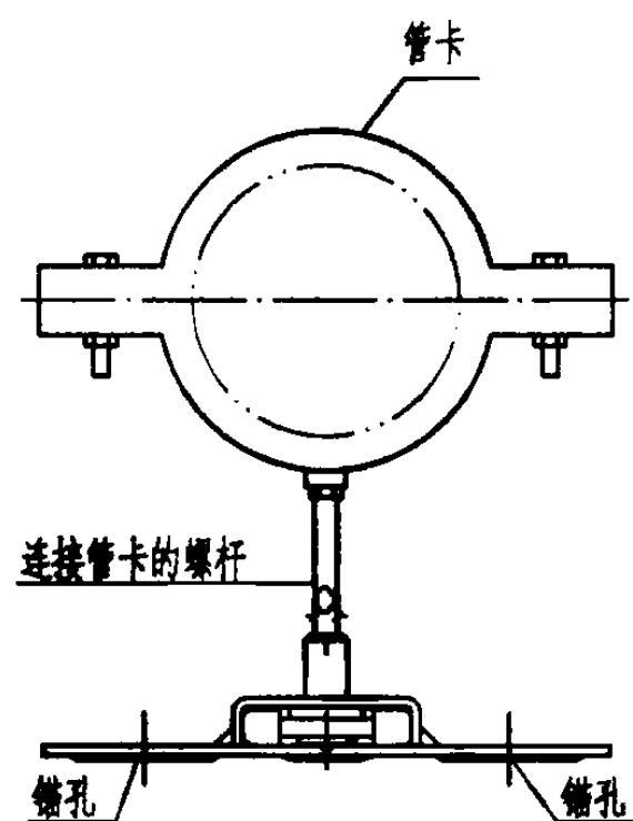
滑动支座MSG1.0正立面
