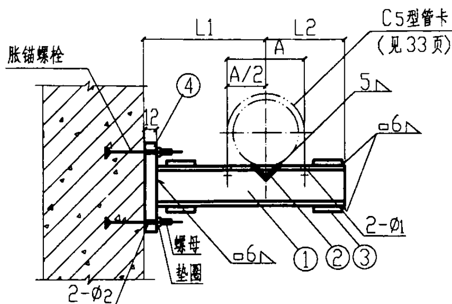
立面图(平面图)
