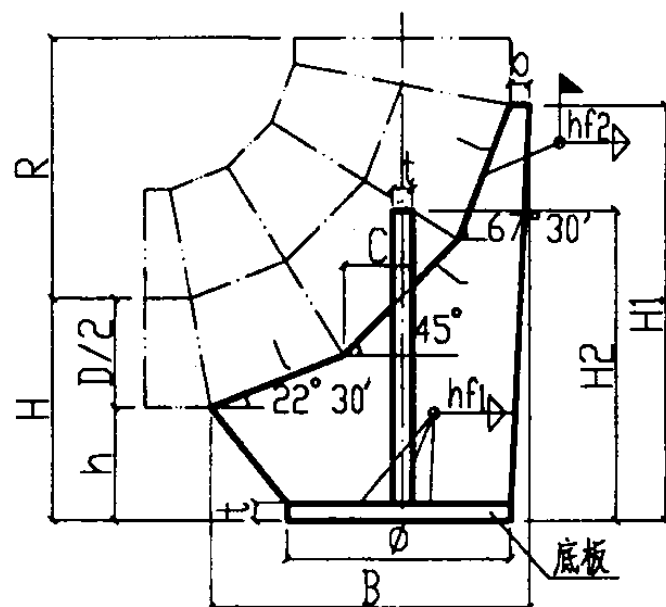
DN450-DN500立面图
