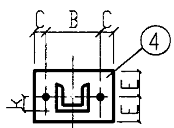
钢板大样图
