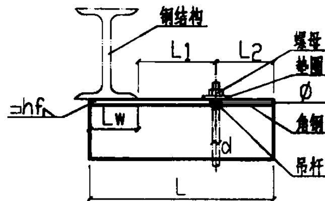
立面图
