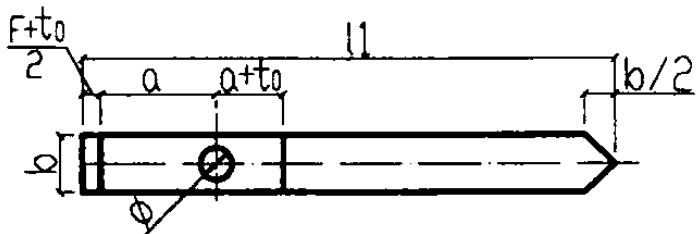
卡板一展开图
