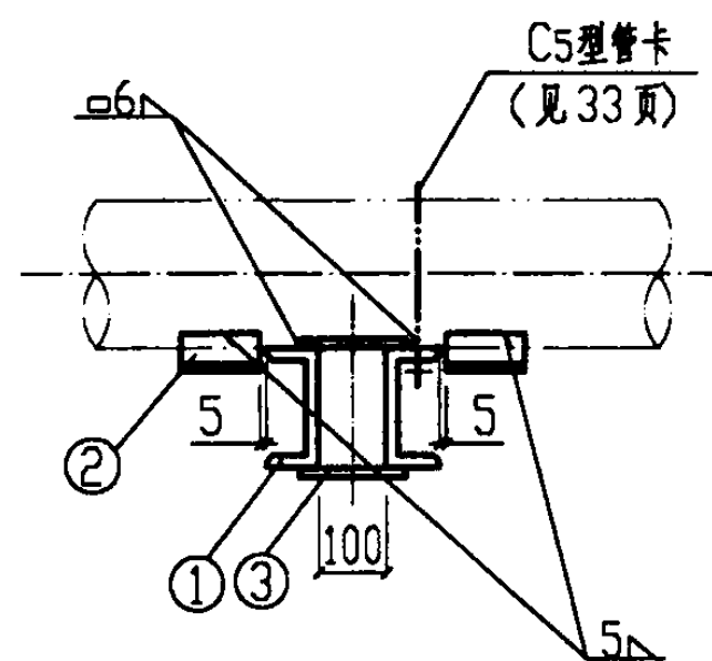
I-I视图
