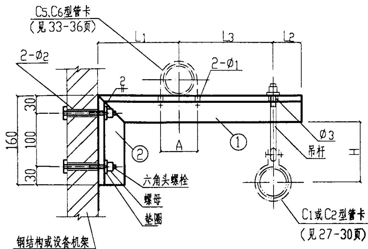
立面图
