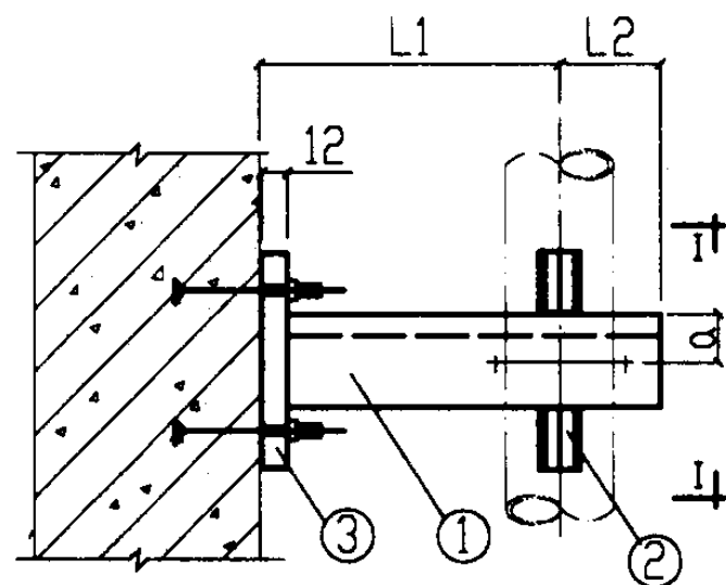
平面图(立面图)
