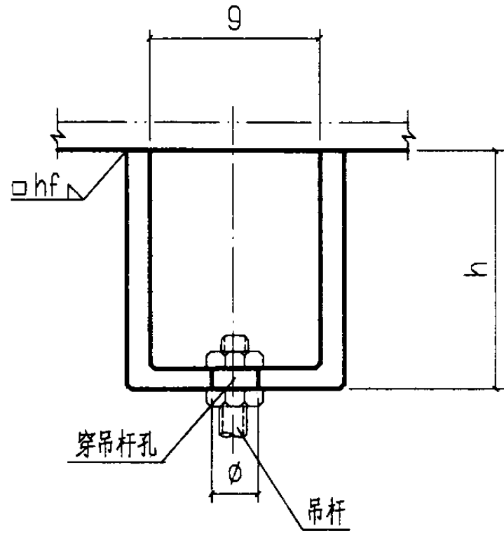
立面图
