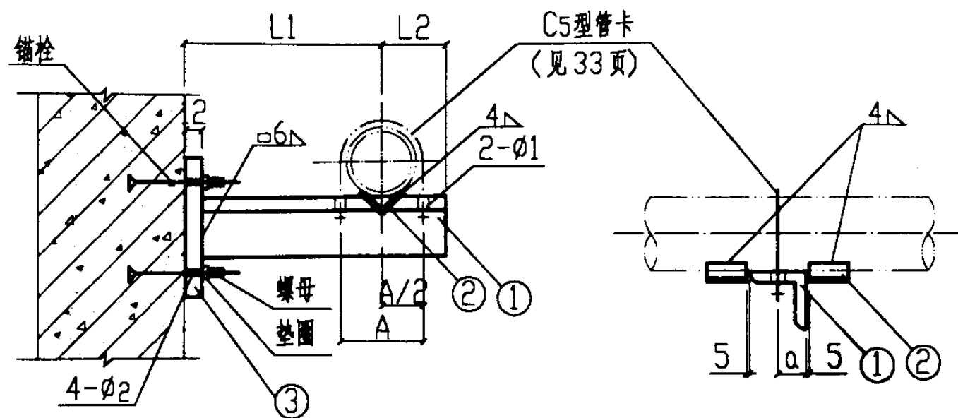
I-I视图
