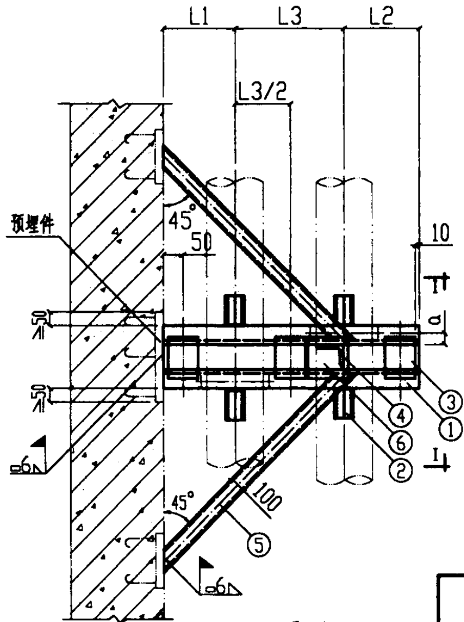
平面图
