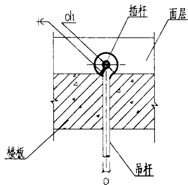
立面图
