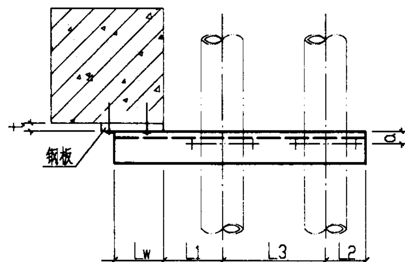
平面图
