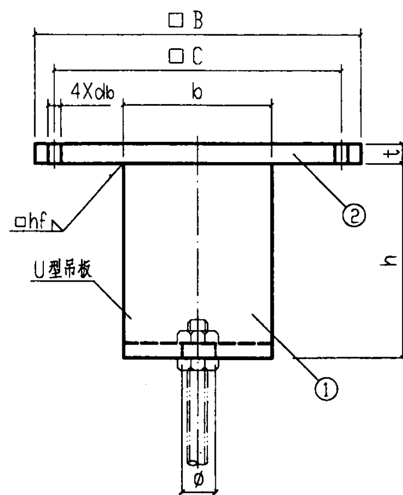
側面圖
