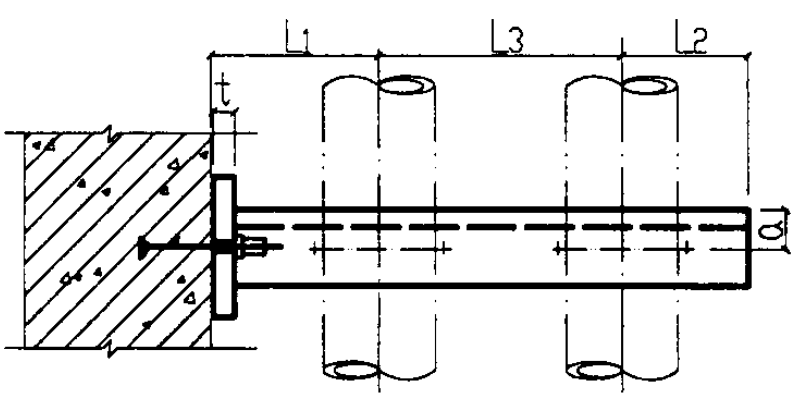
平面图
