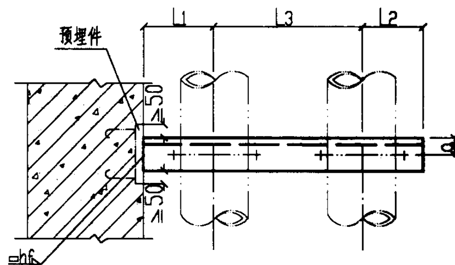
平面图
