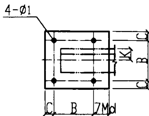
钢板大样图
