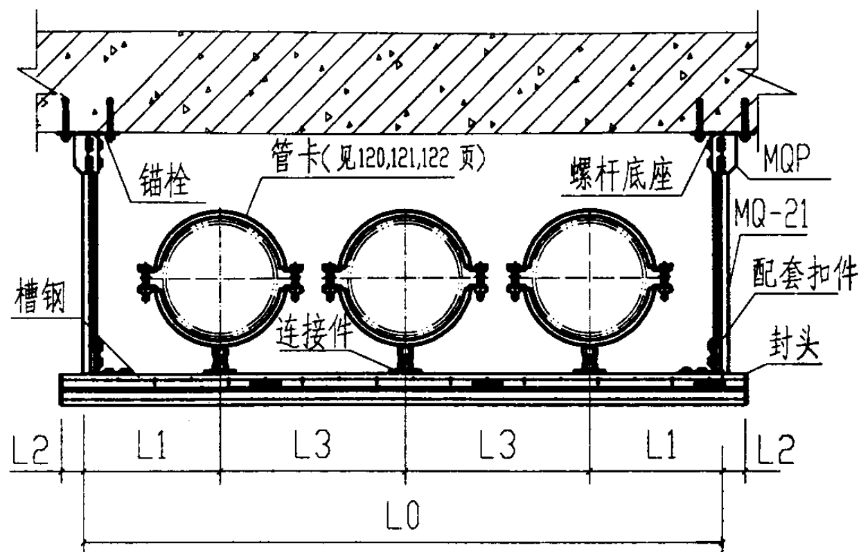
立面图
