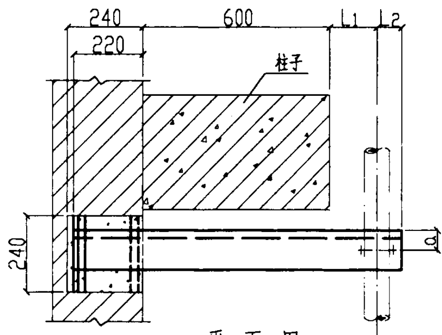
平面图
