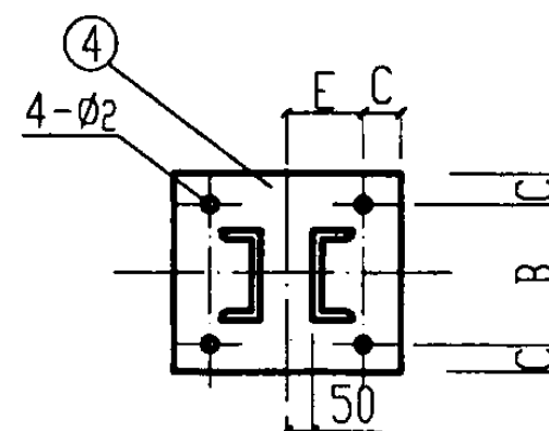
钢板大样图
