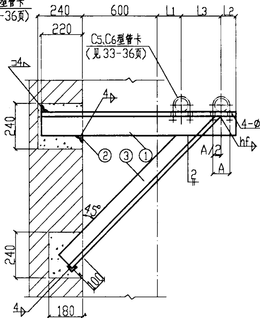
DN65-DN100 立面图
