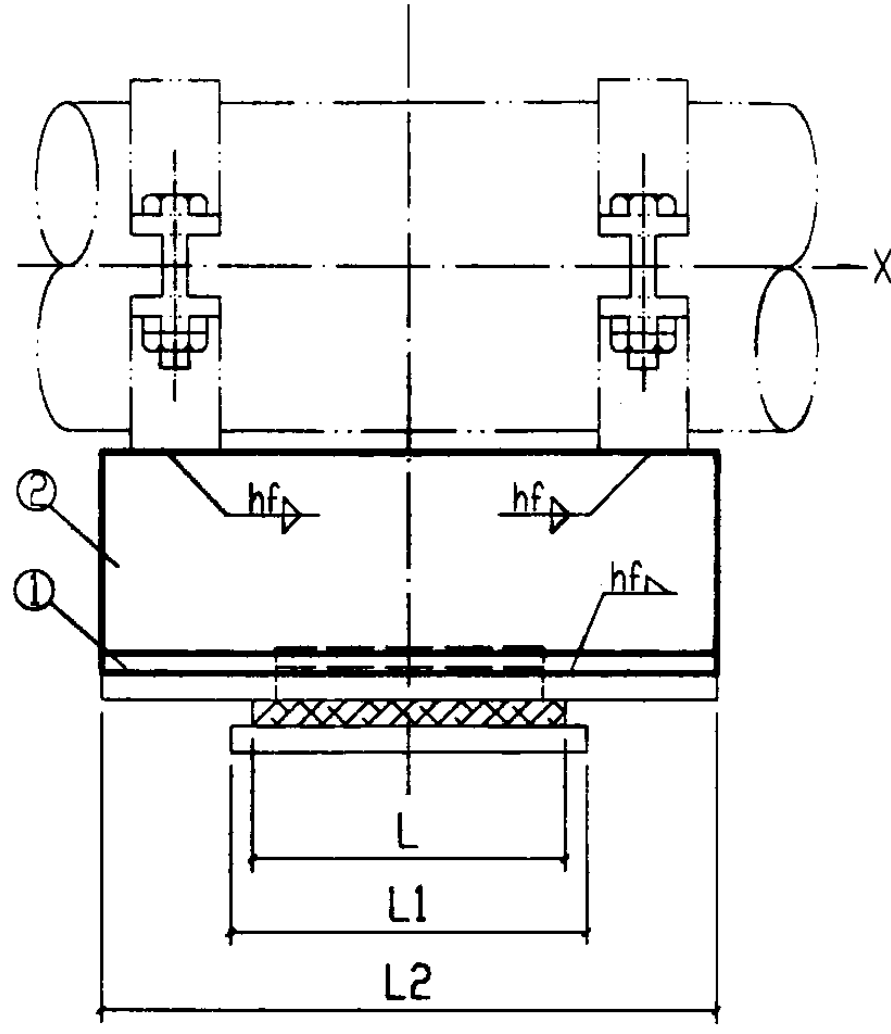
立面图
