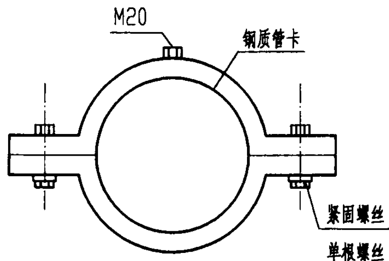
类型11 MFP-L-NW
