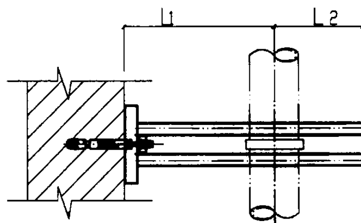
平 面 图
