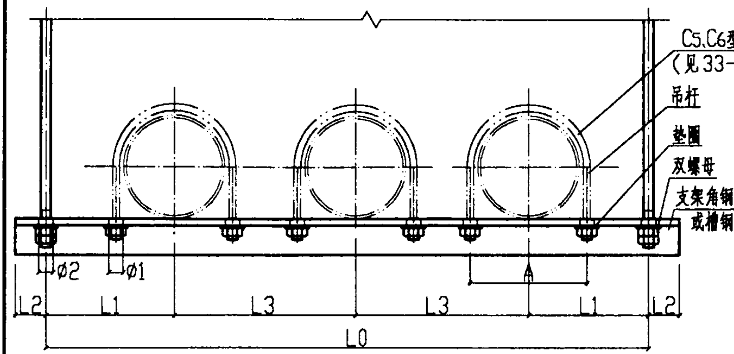
立面图
