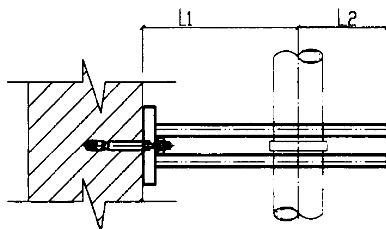
平面图
