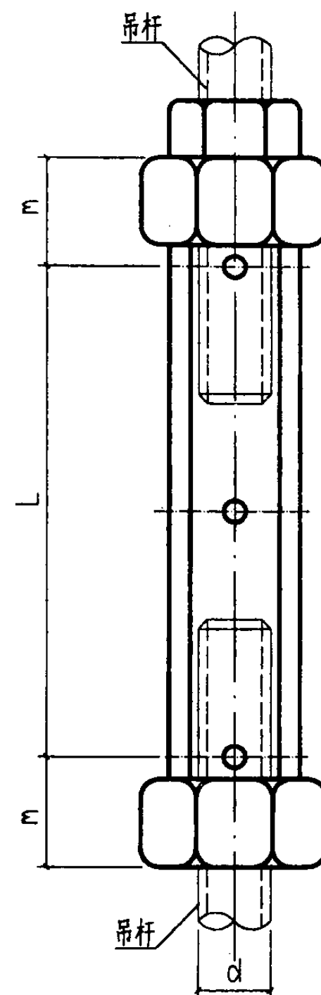
长型螺旋扣
