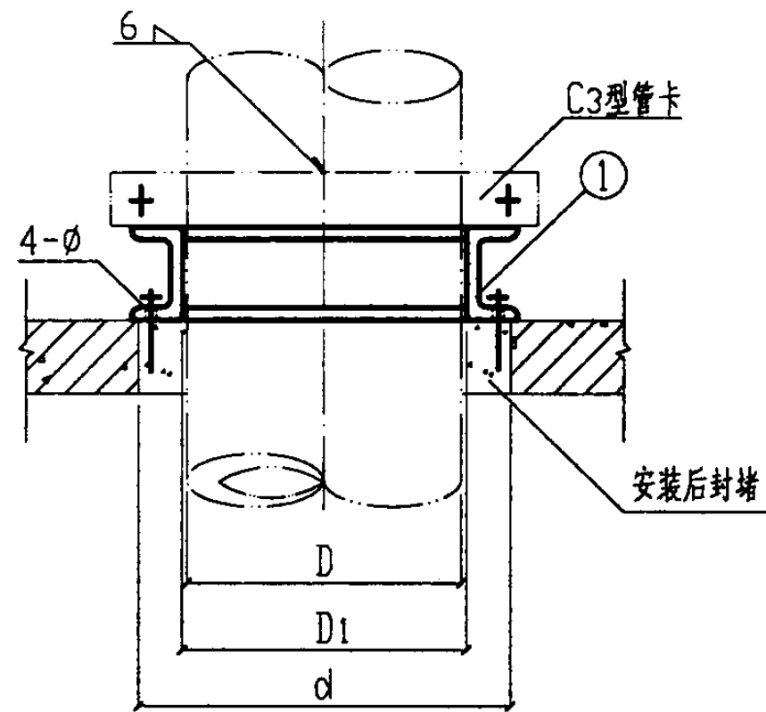
立面图
