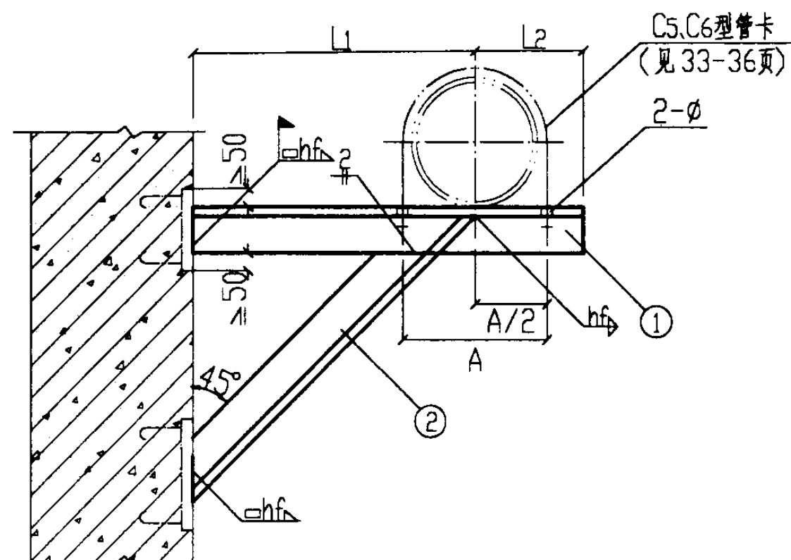
立视图
