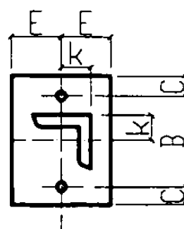
钢板大样图
