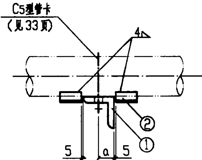
I-I视图
