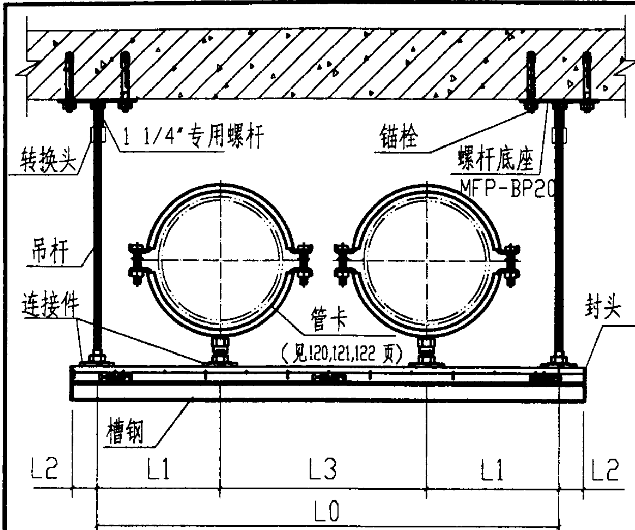
立面图
