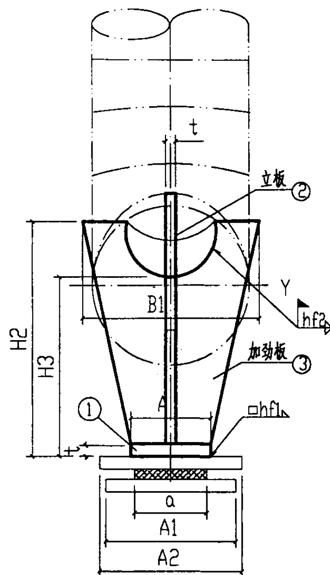
侧面图
