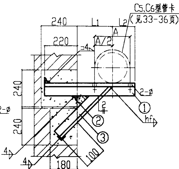
DN200-DN300 立面图
