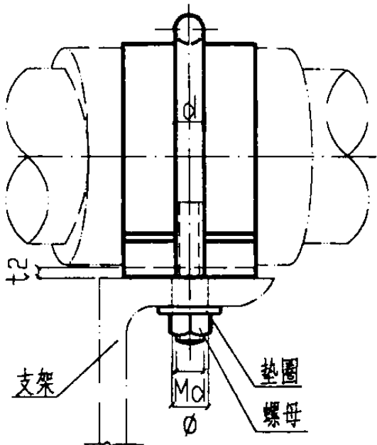
侧面图
