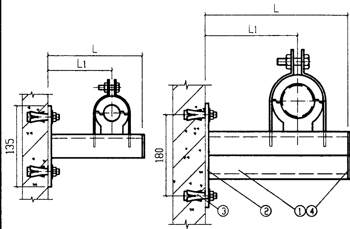
立面图
