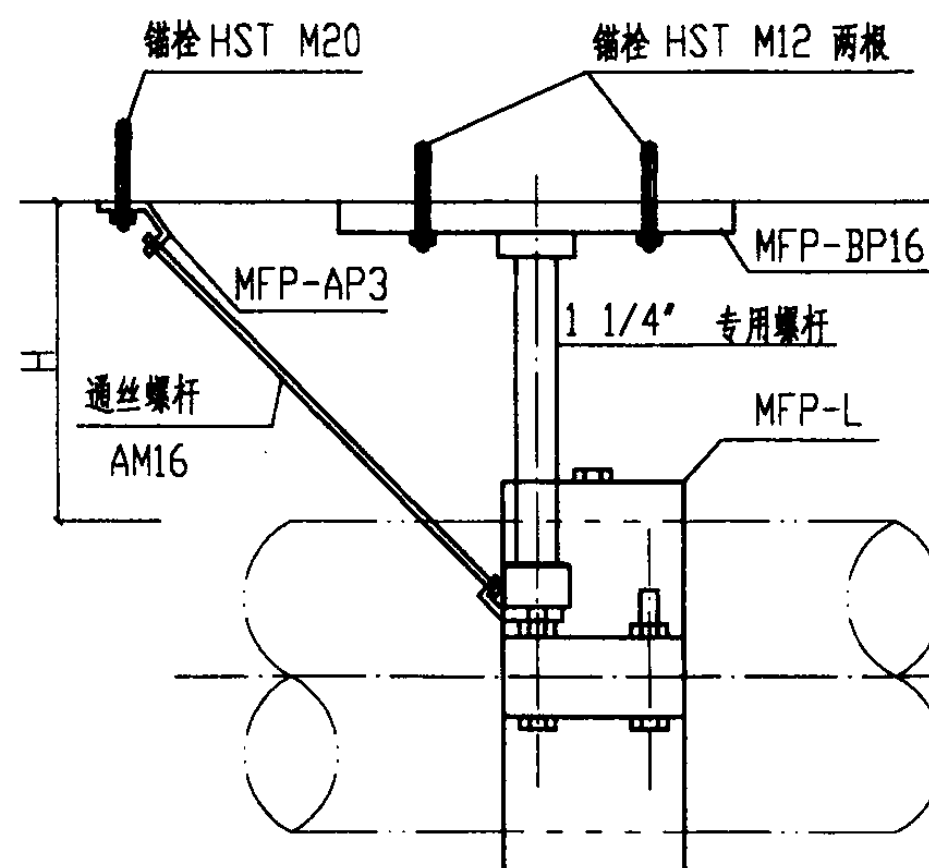
类型4 MFP3固定支座侧立面
