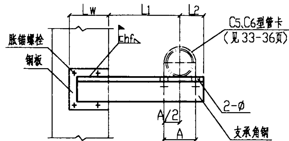
立面图
