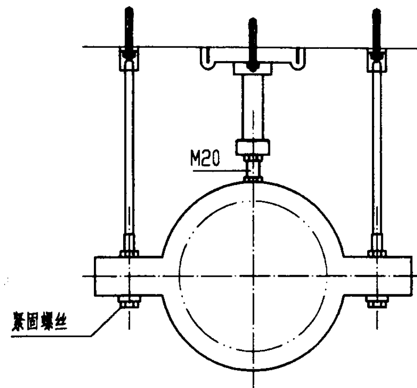
类型3 MFP2固定支座正立面
