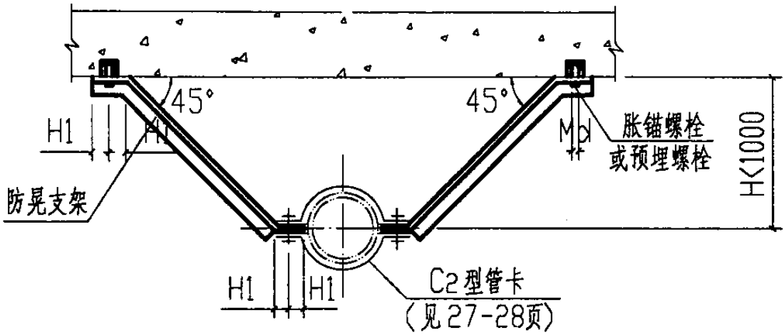
立面图
