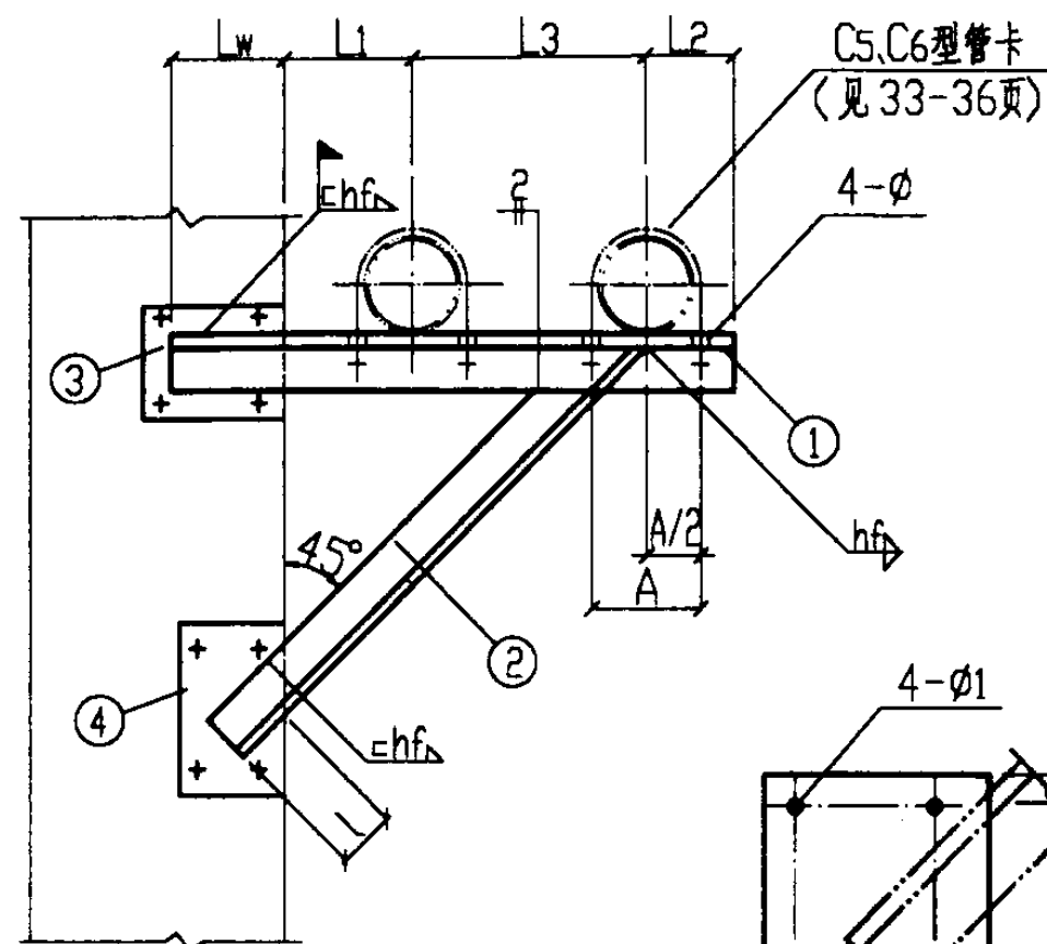
立面图
