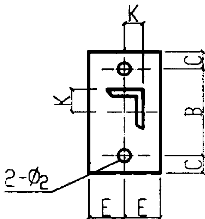
钢板大样图
