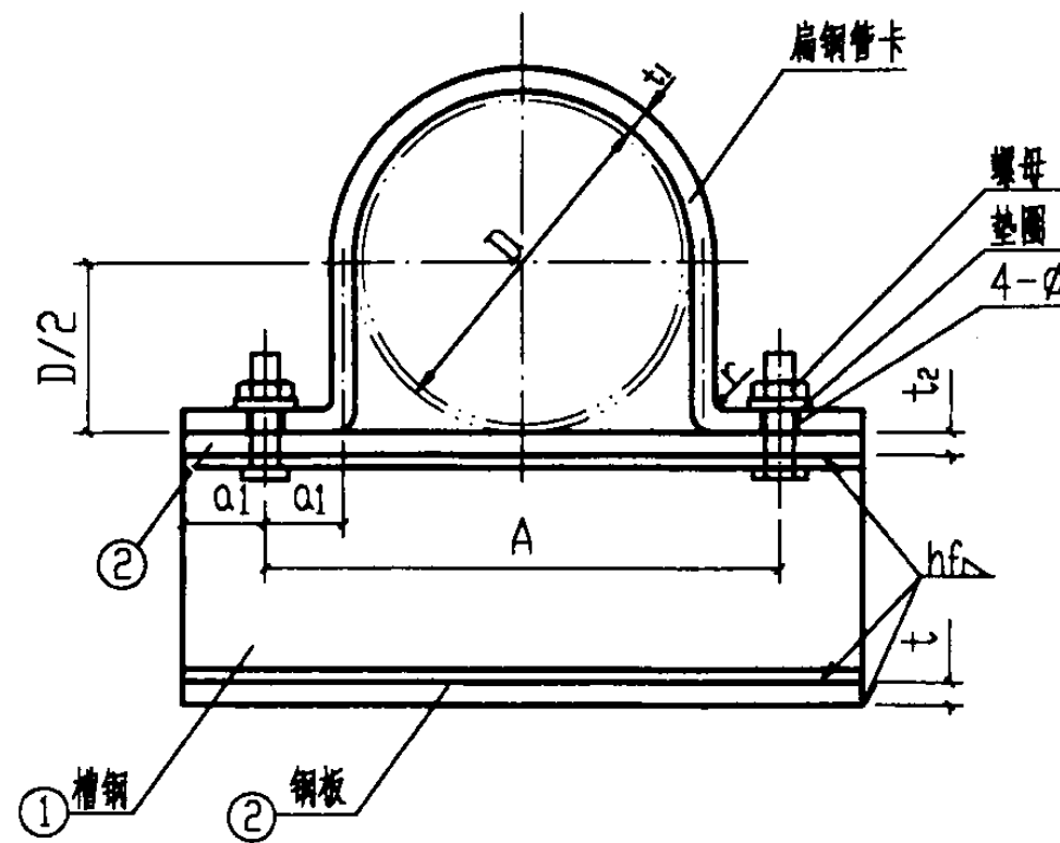
立面图
