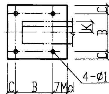
钢板大样图
