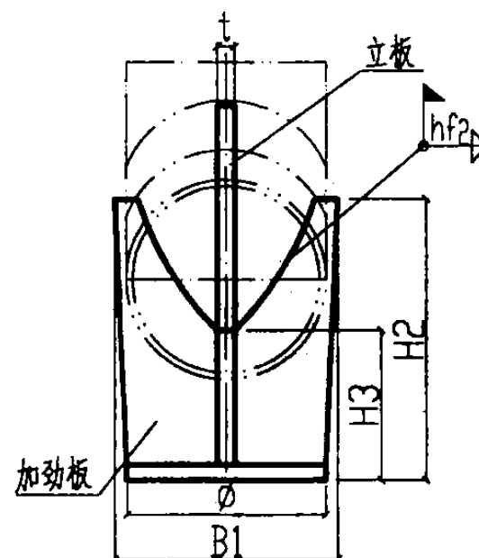
DN450-DN500侧面图
