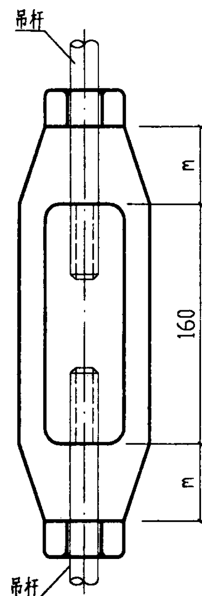
短型螺旋扣
