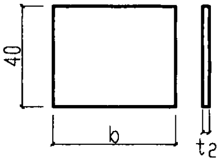
钢弧形板展开图
