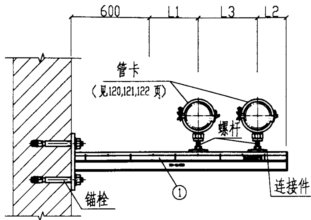
DN15-50 立面图
