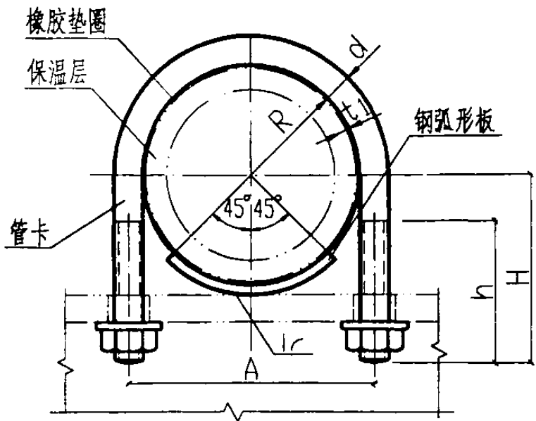
立面图
