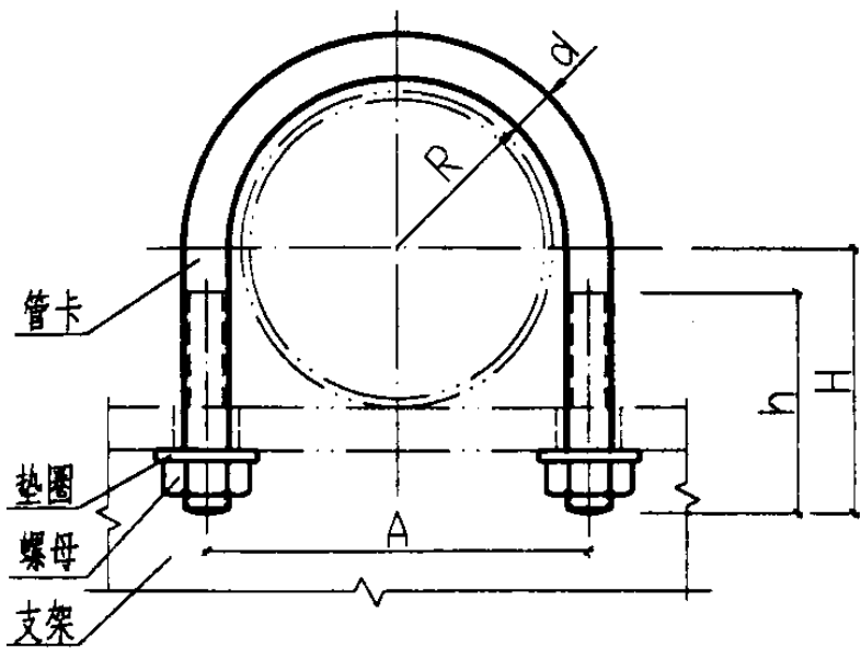
立面图
