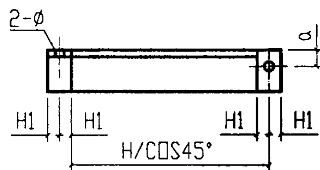
防晃支架展开图
