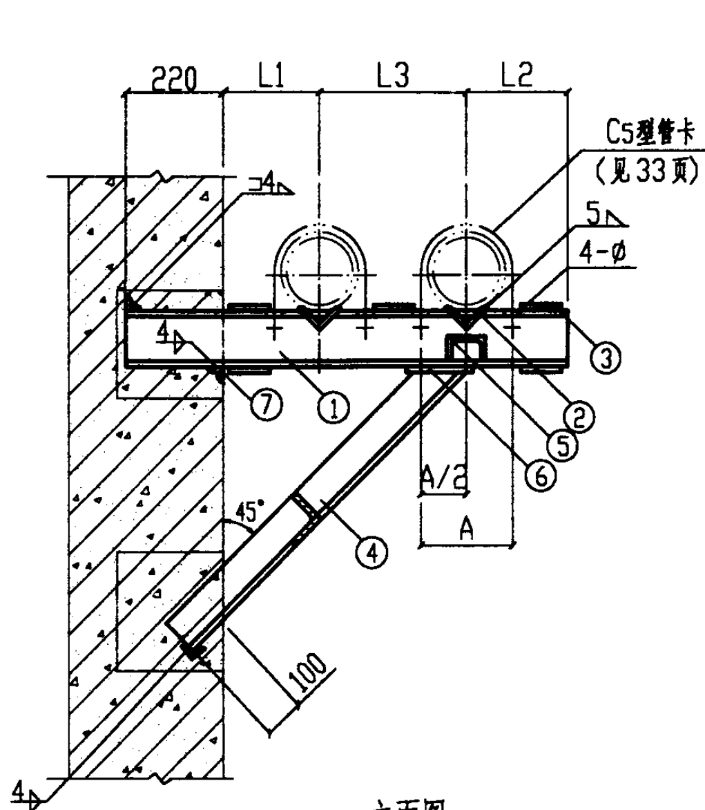
立面图
