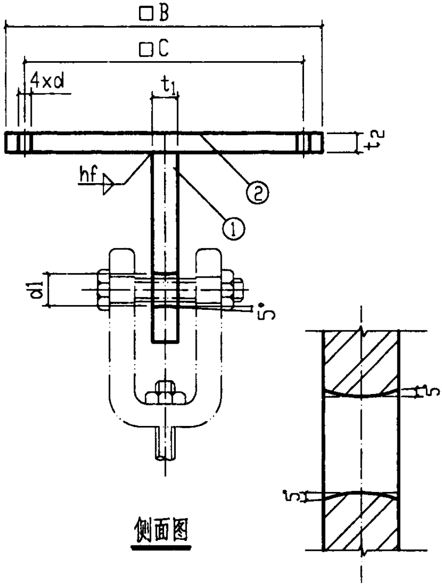
双锥形孔大样图
