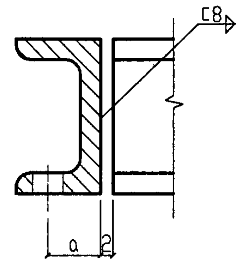
A-A 剖面图
