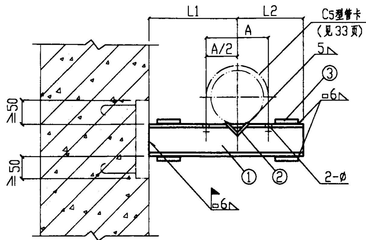
立面图 (平面图)
