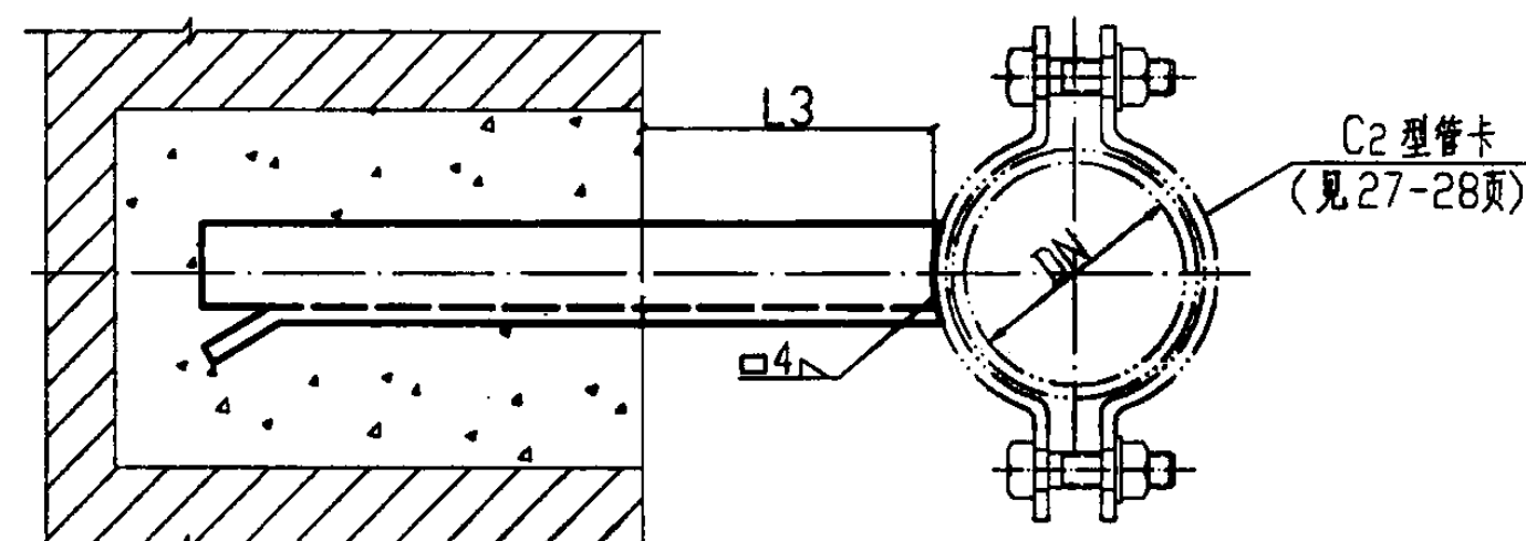
平面图
