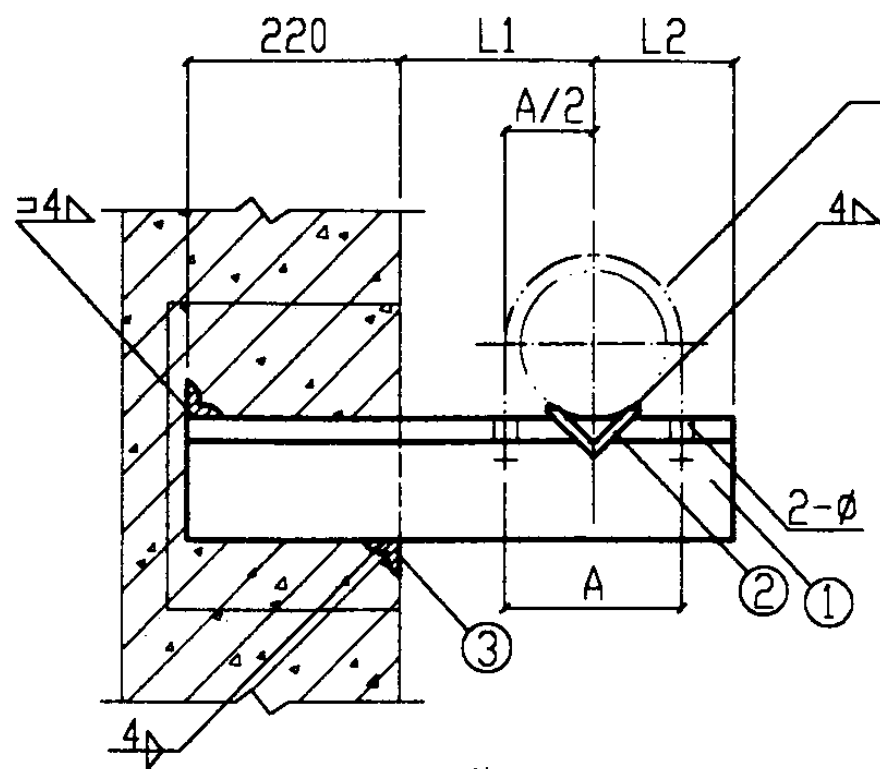
立面图 (平面图)
