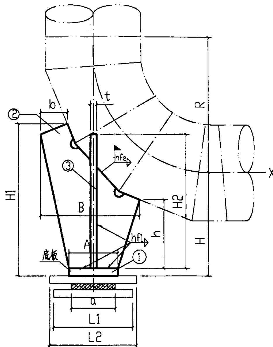
立面图
