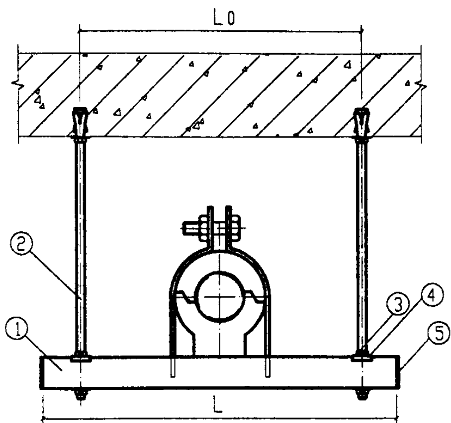
立面图(保温)
