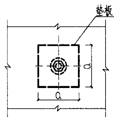
平面图
