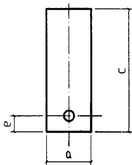
梁夹展开图
