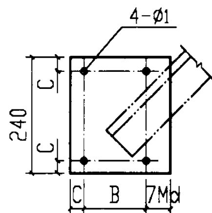
钢板④大样图
