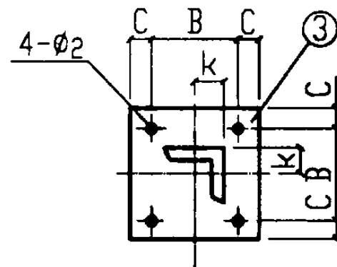
钢板大样图
