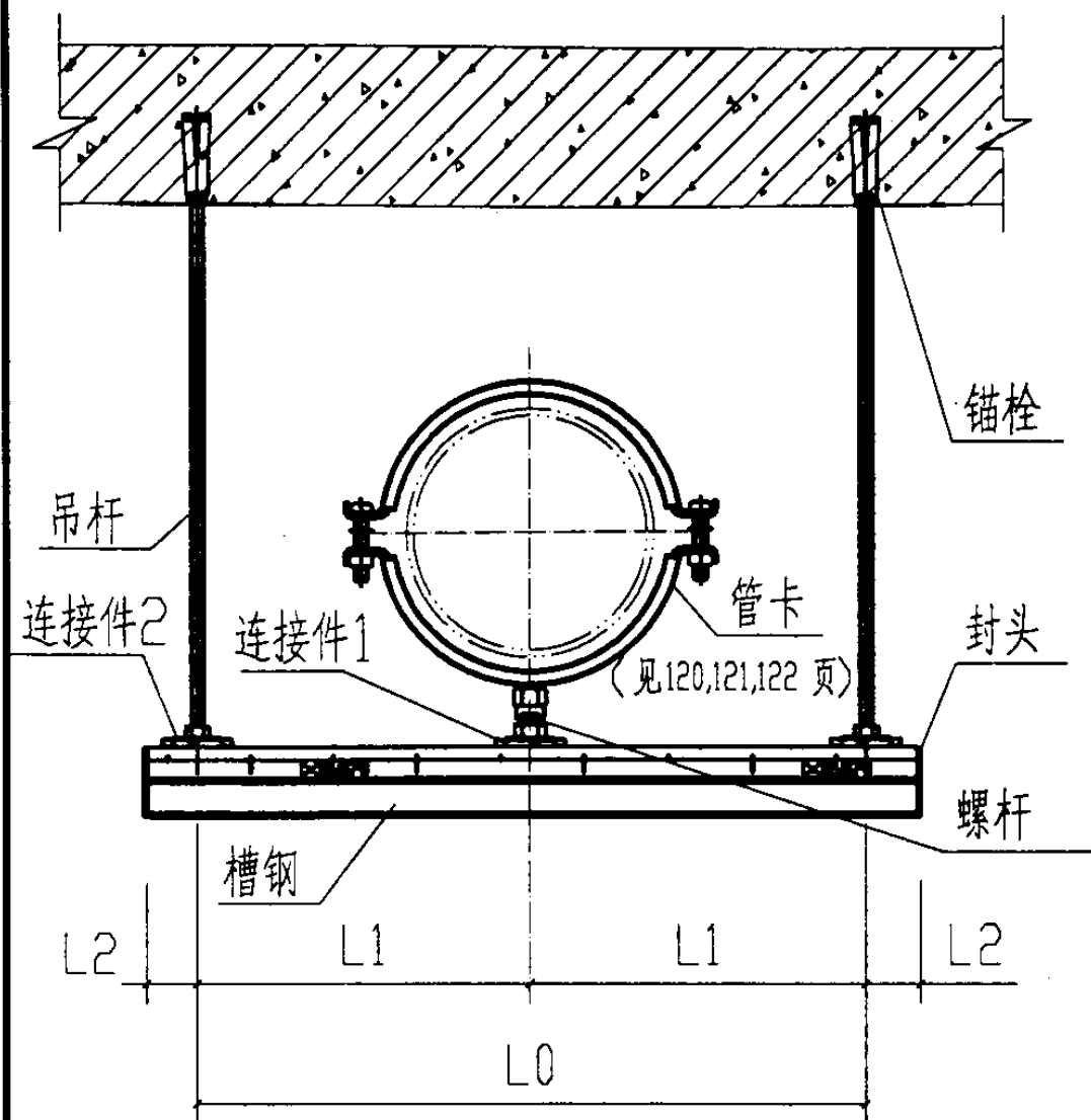
立面图
