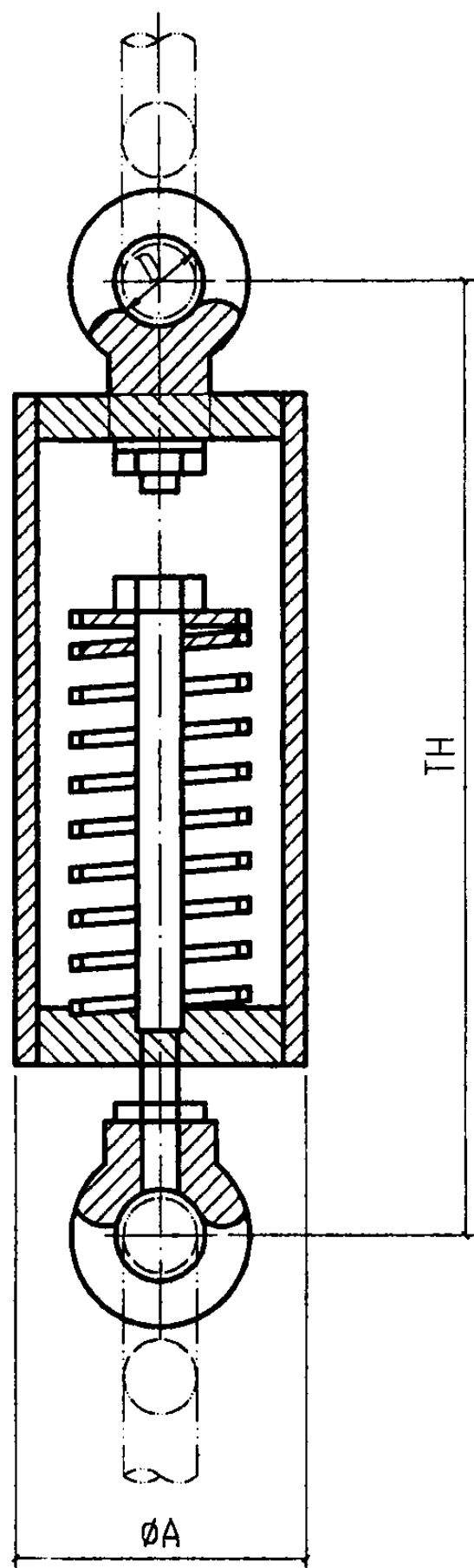
弹簧吊架示意图
