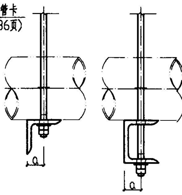
侧面图 槽钢a值位置图
