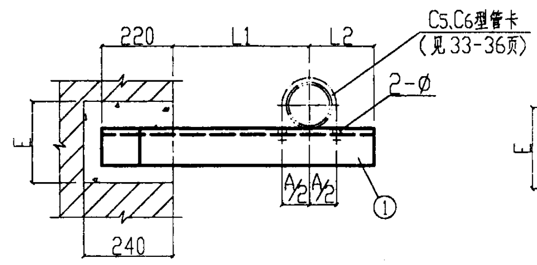
DN50-DN150 平面图
