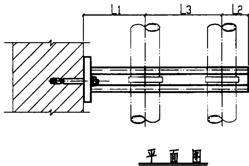
尺寸表
