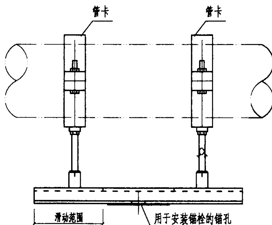
滑动支座MSG1.0侧立面
