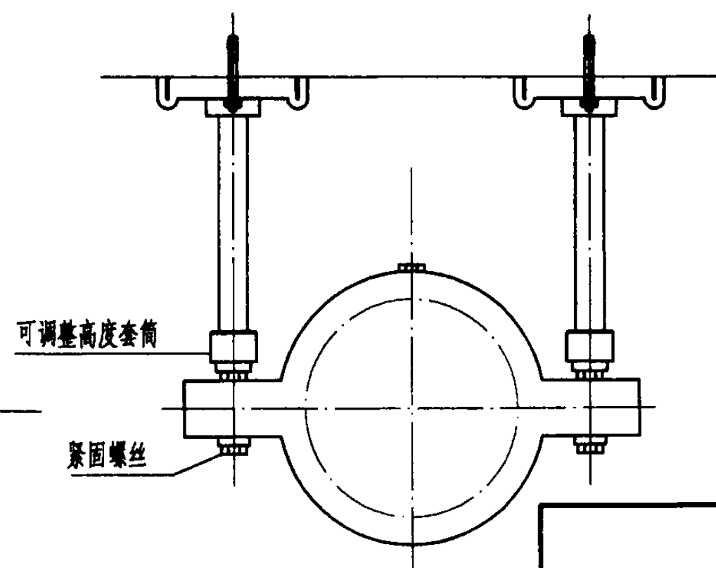
类型4 MFP3固定支座正立面
