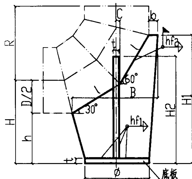
DN200-DN400立面图
