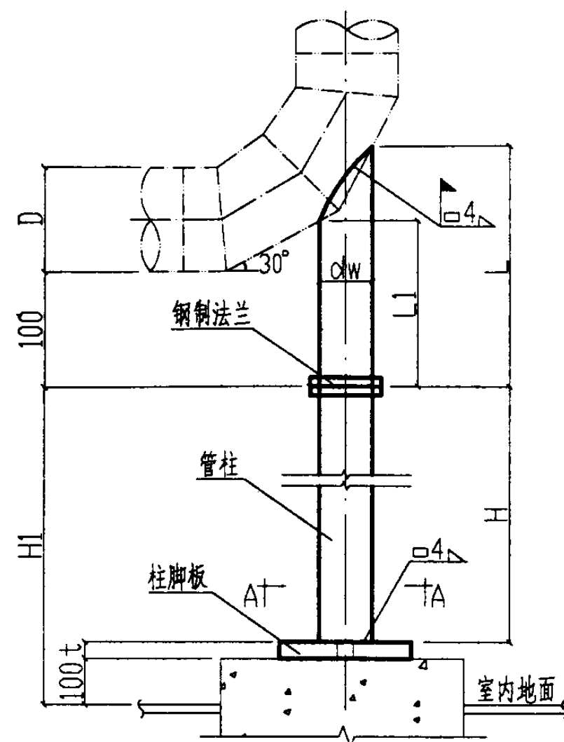
DN100-DN400 立面图
