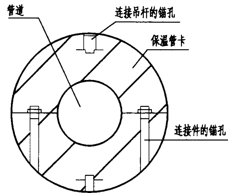
类型9 KF175
