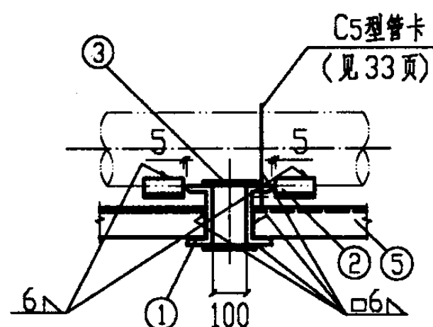
I-I 视图
