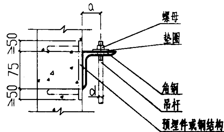
侧面图
