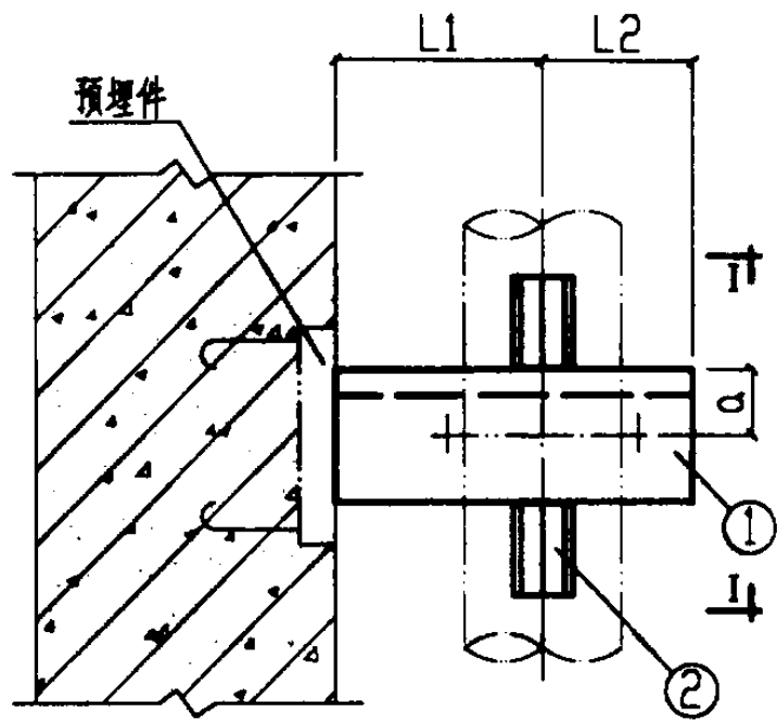
平面图 (立面图)
