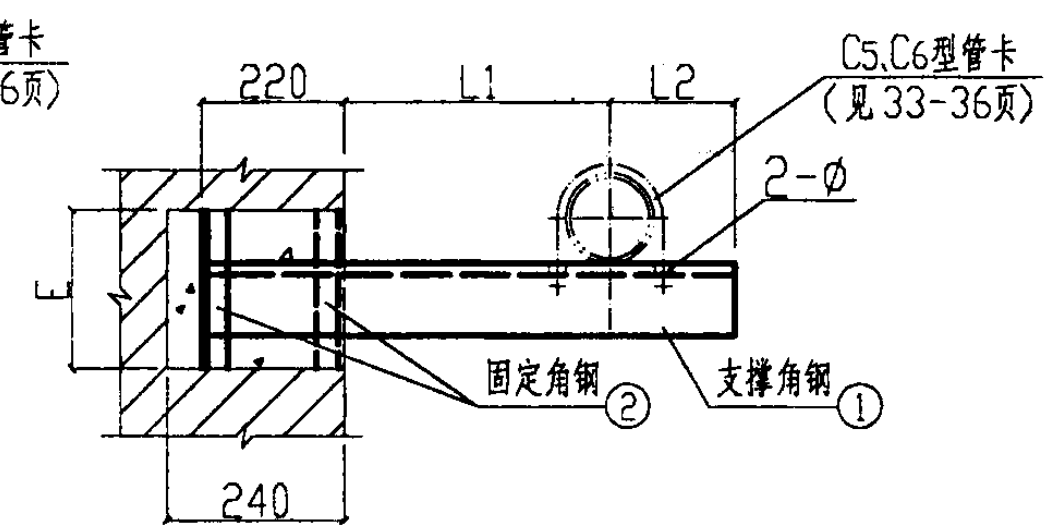
DN200-DN400 平面图
