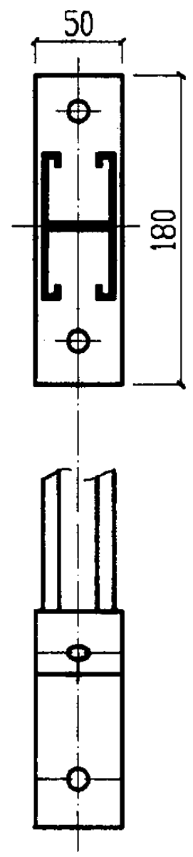
A-A剖面图
