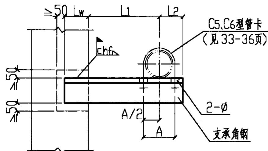
立面图
