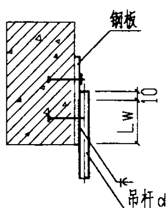
侧面图
