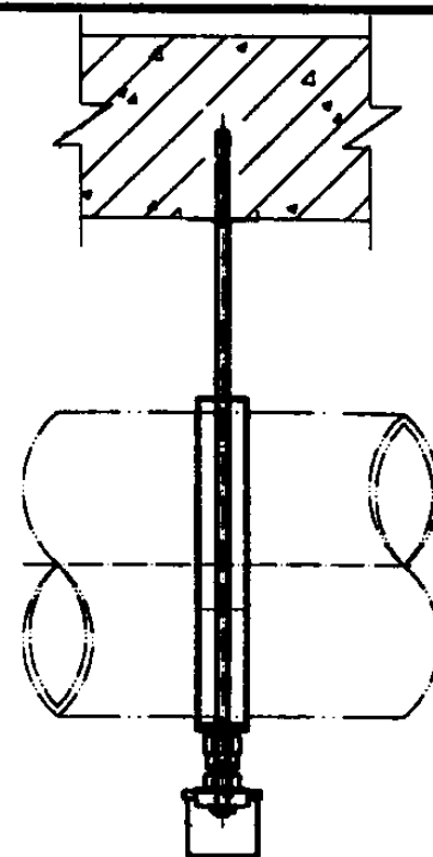
侧面图
