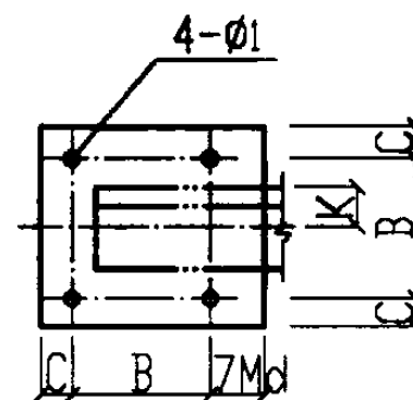
钢板③大样图
