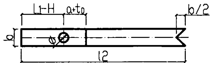
I型卡板二展开图
