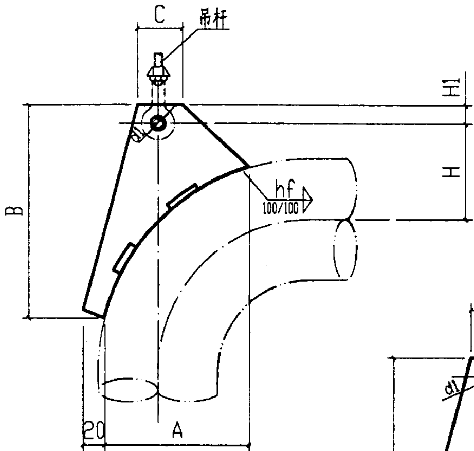
立 面 图
