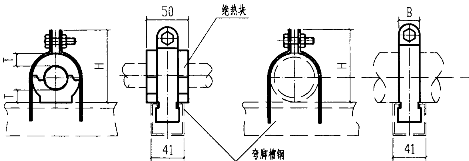
立面图 (保温) 侧面图
