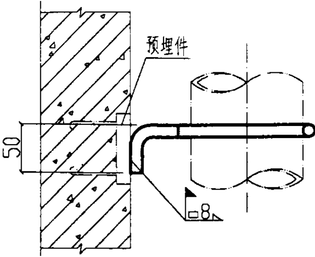
I型立面图
