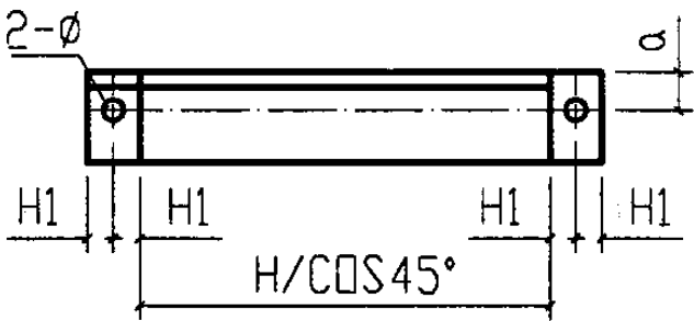
防晃支架展开图
