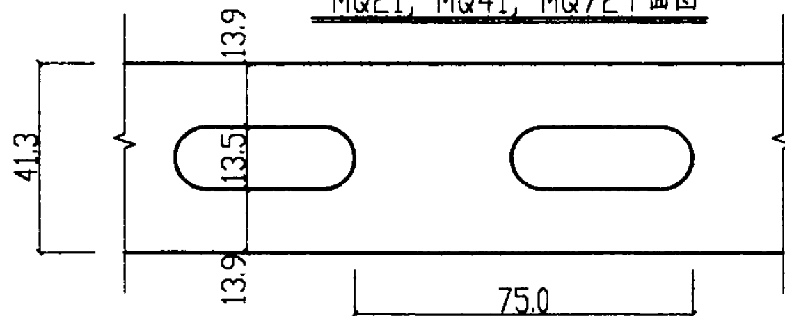
MQ21D, MQ41D, MQ-52-72D, MQ-124XD平面图
