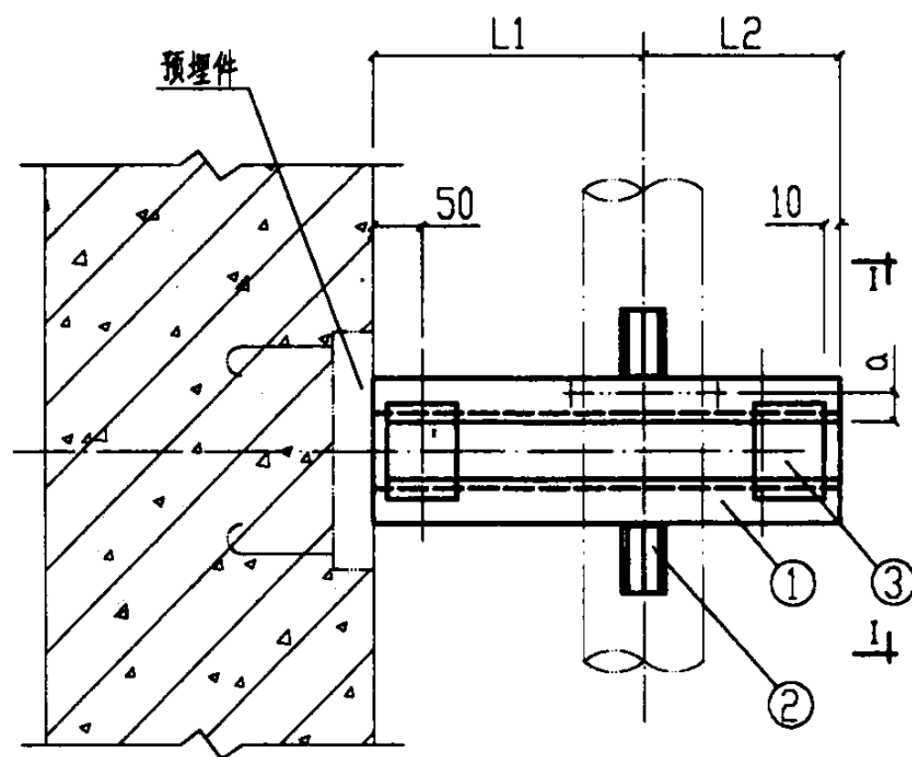
平面图 (立面图)
