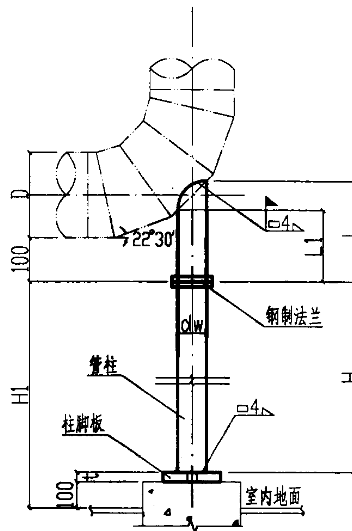
DN450-DN500 立面图
