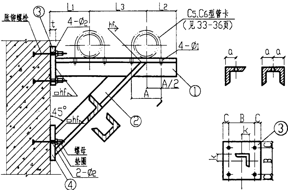
立面图
