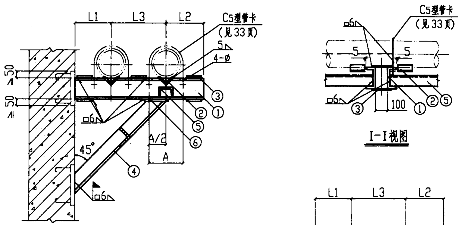
立面图
