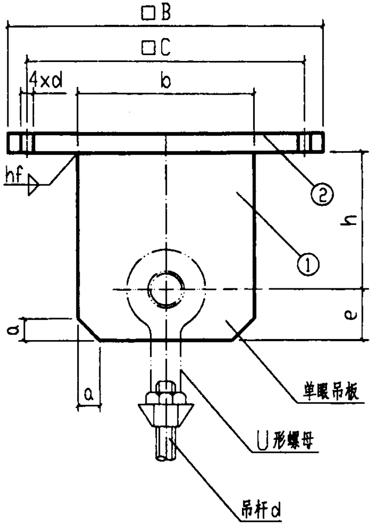
立面图
