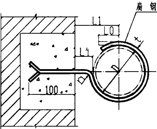
II型平面图
