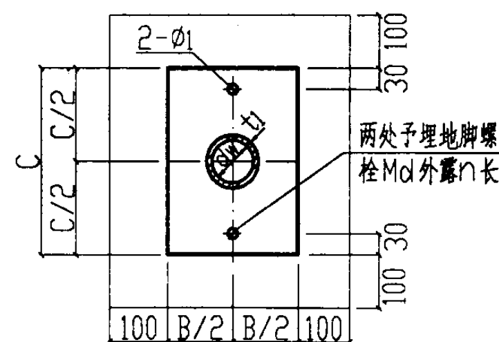
A-A剖面图
