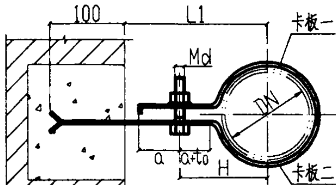
II型支架平面图
