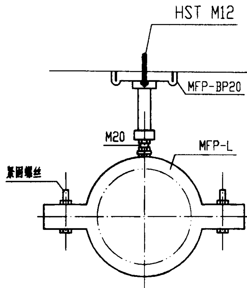
类型1 MFP1固定支座正立面
