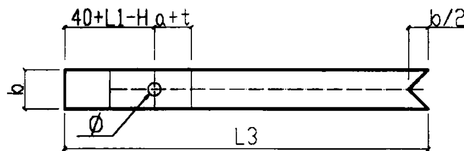
卡板二展开图
