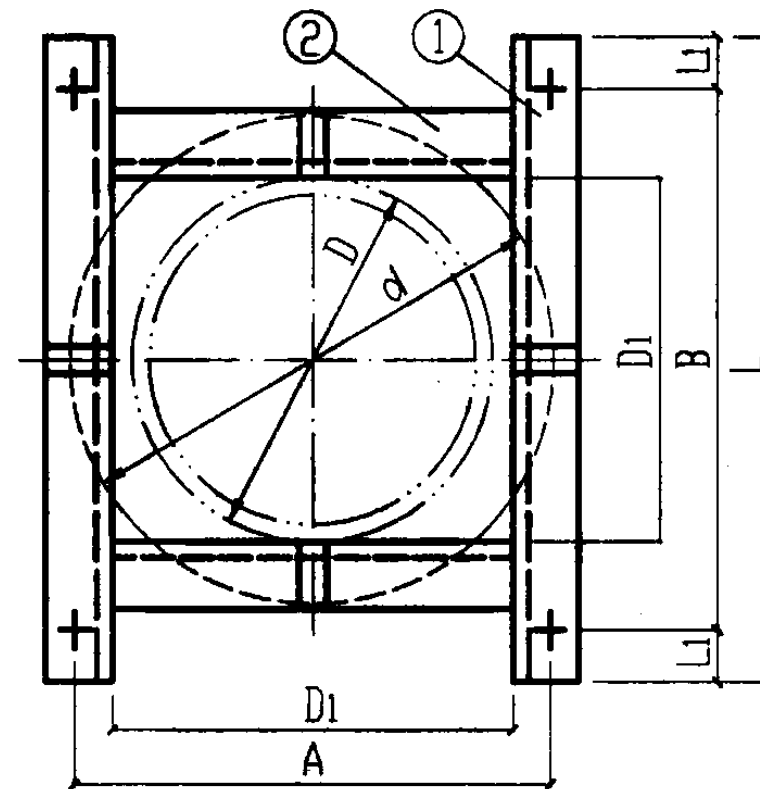
平面图
