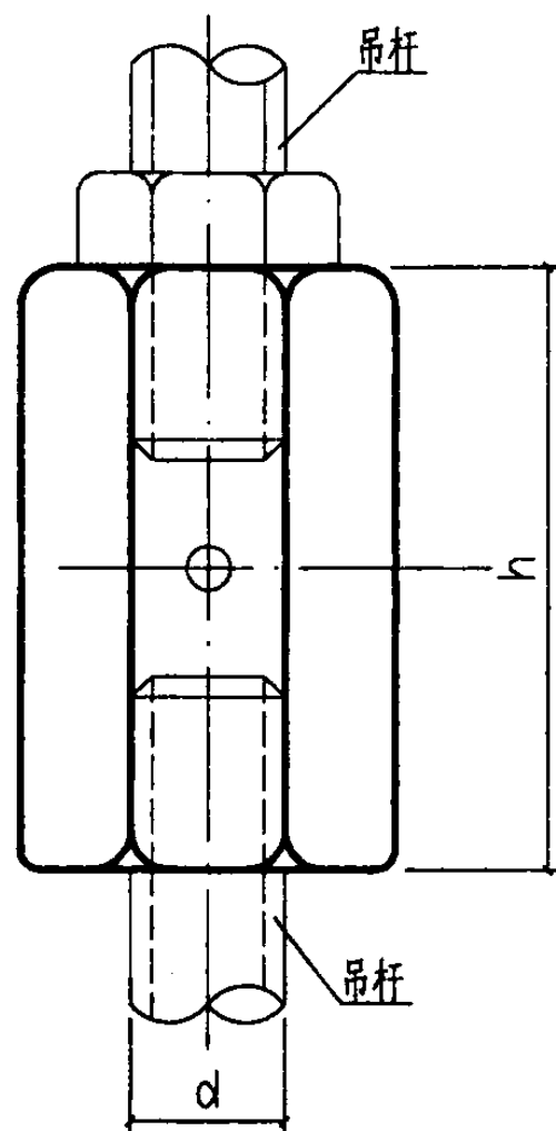
等径连接螺母
