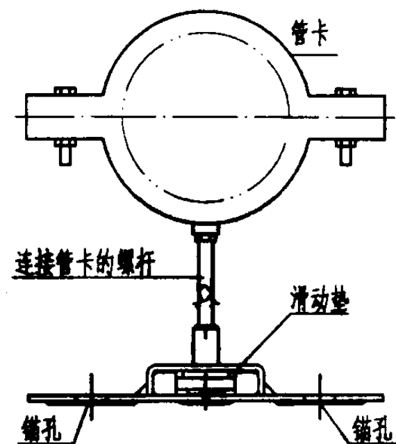
滑动支座MSG1.0正立面
